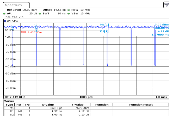
11G_Ant1_2442
