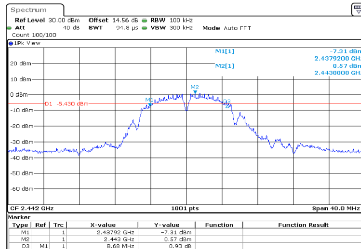
11B_Ant1_2442
