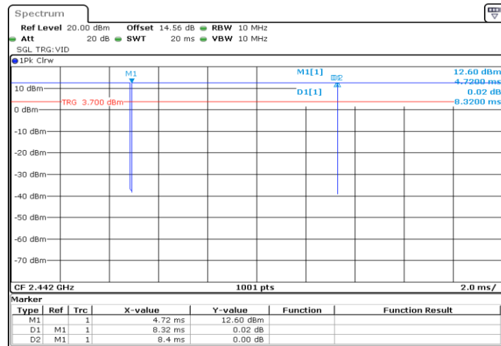
11B_Ant1_2442
