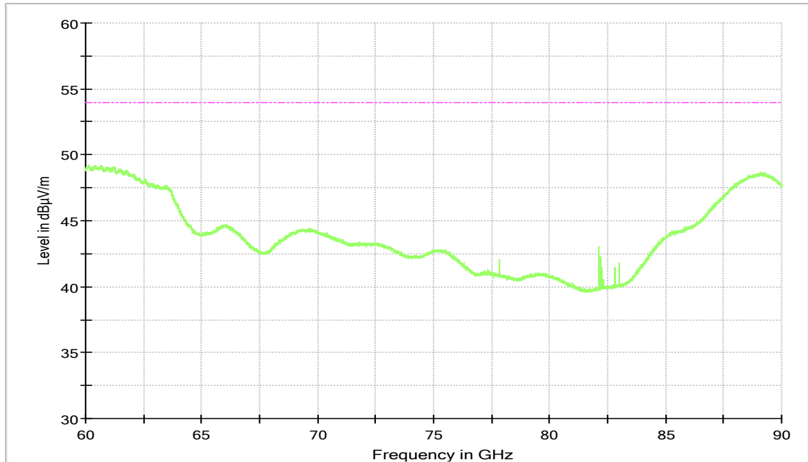
S01_AB01 60 GHz – 90 GHz
