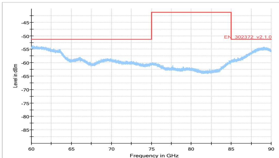
S01_AB01 60 GHz – 90 GHz
