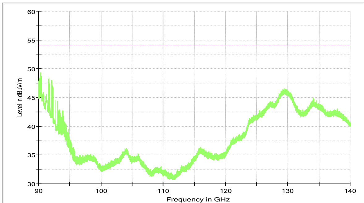
S01_AB01 90 GHz – 140 GHz
