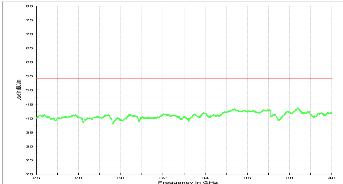
S01_AB01 26 GHz – 40 GHz
