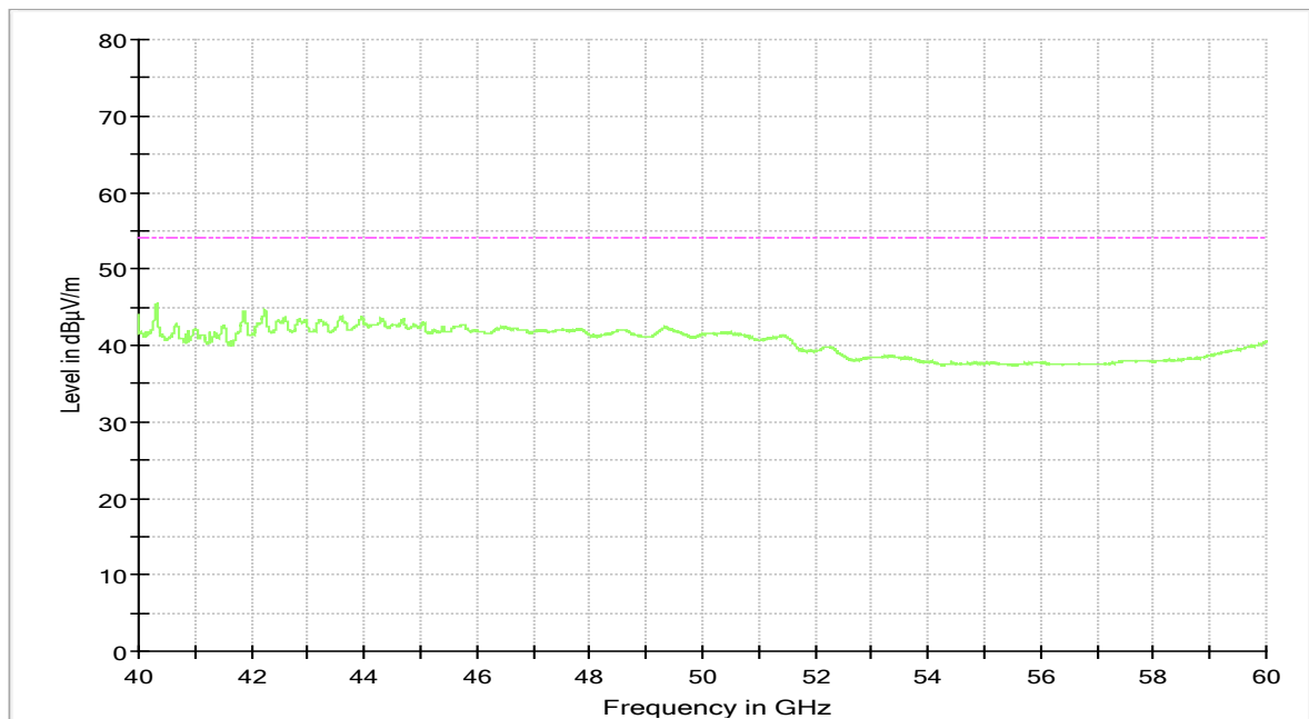
S01_AB01 40 GHz – 60 GHz
