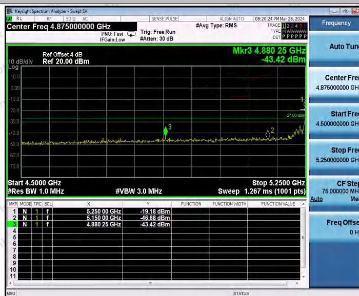
11AC80MIMO_Ant1_Low_5290
