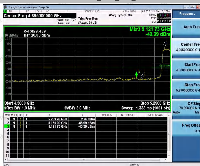
11AX40MIMO_Ant2_Low_5270
