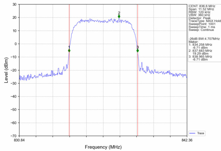
Band5_HSUPA_MCH_836.6MHz_Subtest 1_NTNV
