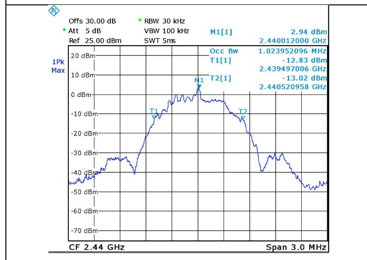
Figure 17. 2440.0 MHz, BLE
