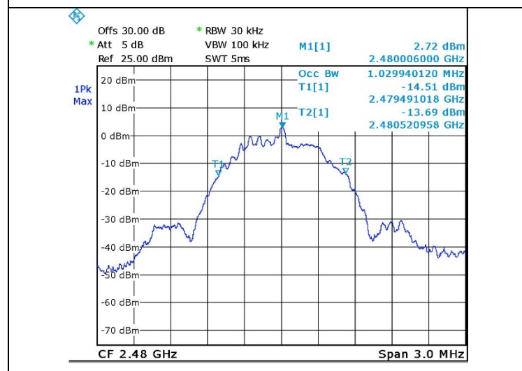
Figure 18. 2480.0 MHz, BLE
