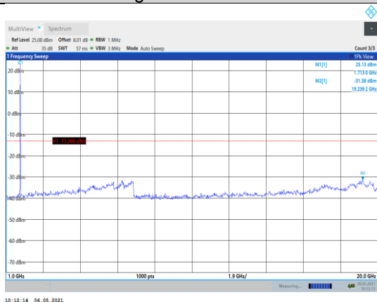
Band4-3MHz-QPSK-19965-1RB#0- Range2:1000~20000MHz
