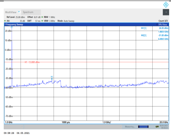
Band2-20MHz-16QAM-18900-1RB#0- Range2:1000~20000MHz
