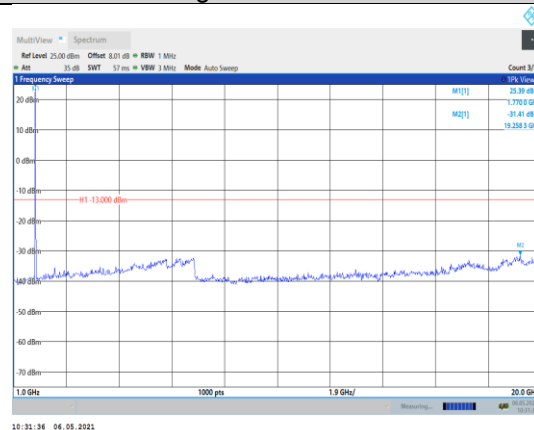
Band66-5MHz-QPSK-132647-1RB#0- Range2:1000~20000MHz
