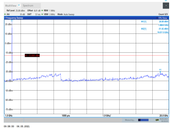
Band2-20MHz-QPSK-19100-1RB#0- Range2:1000~20000MHz
