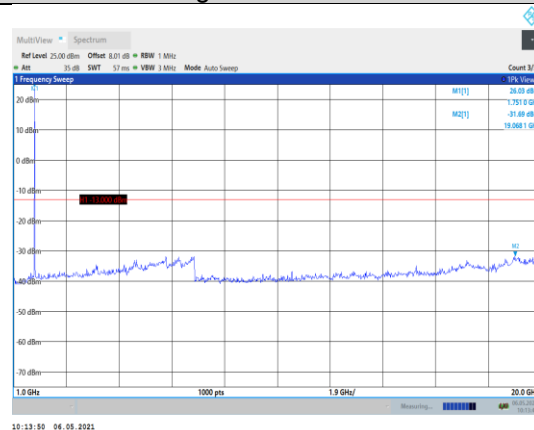
Band4-3MHz-QPSK-20385-1RB#0- Range2:1000~20000MHz
