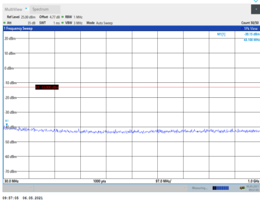
Band2-20MHz-QPSK-18700-1RB#0- Range1:30~1000MHz
