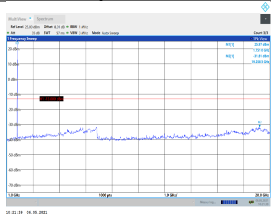
Band4-1.4MHz-QPSK-20393-1RB#0- Range2:1000~20000MHz
