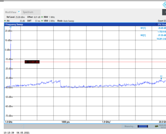
Band4-10MHz-QPSK-20175-1RB#0- Range2:1000~20000MHz
