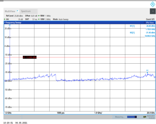
Band4-1.4MHz-QPSK-20175-1RB#0- Range2:1000~20000MHz
