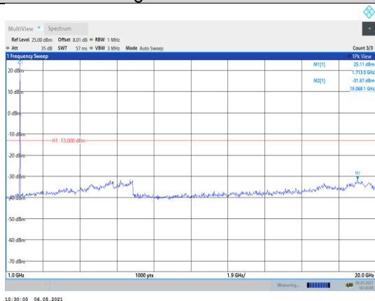
Band66-5MHz-QPSK-131997-1RB#0- Range2:1000~20000MHz
