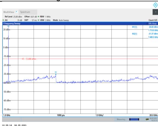
Band66-3MHz-QPSK-131987-1RB#0- Range2:1000~20000MHz
