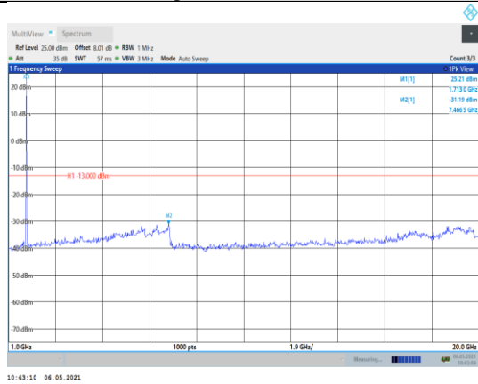
Band66-10MHz-QPSK-132022-1RB#0- Range2:1000~20000MHz
