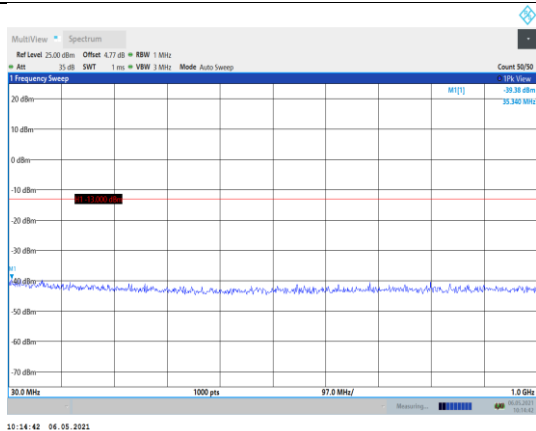
Band4-10MHz-QPSK-20000-1RB#0- Range1:30~1000MHz
