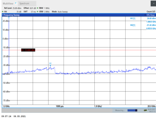
Band2-20MHz-QPSK-18700-1RB#0- Range2:1000~20000MHz
