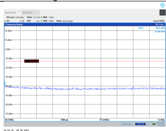
Band4-1.4MHz-QPSK-20393-1RB#0- Range1:30~1000MHz
