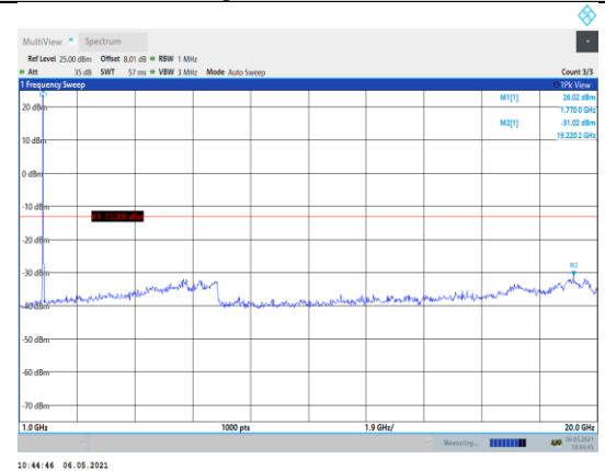
Band66-10MHz-QPSK-132622-1RB#0- Range2:1000~20000MHz
