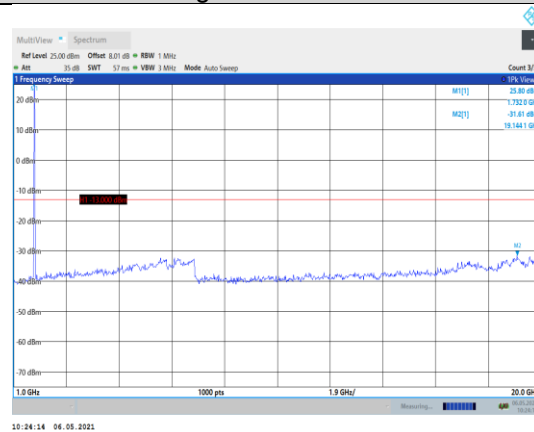
Band4-15MHz-QPSK-20325-1RB#0- Range2:1000~20000MHz
