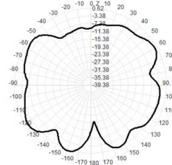
2400.0MHz Total(E2-YZ), Max= -0.63dBi
