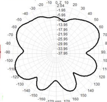
2500.0MHz Total(E1-XZ), Max= 2.04dBi
