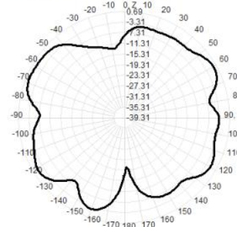
2450.0MHz Total(E2-YZ), Max= -0.61dBi
