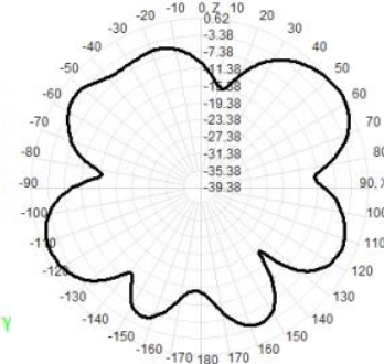
2400.0MHz Total(E1-XZ), Max= 0.62dBi
