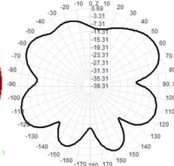
2450.0MHz Total(E1-XZ), Max= 0.69dBi
