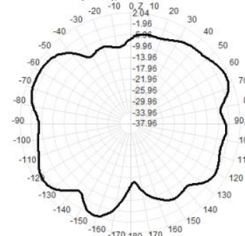
2500.0MHz Total(E2-YZ), Max= 0.68dBi
