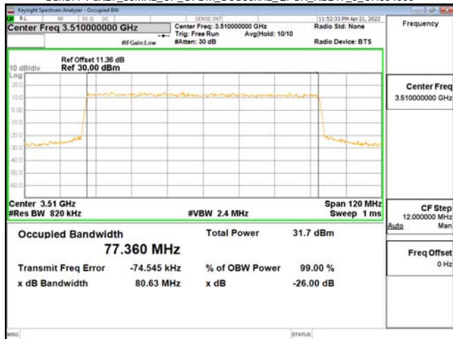
Band77-Part27_80MHz_CP_OFDM_SCS30kHz_QPSK_RB217_0_CH634000
