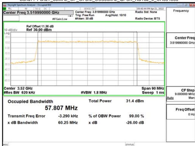
Band77-Part27_60MHz_CP_OFDM_SCS30kHz_QPSK_RB162_0_CH634666
