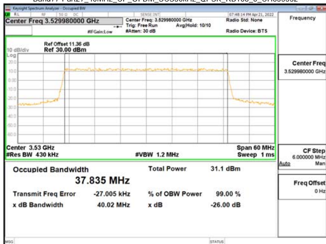
Band77-Part27_40MHz_CP_OFDM_SCS30kHz_QPSK_RB106_0_CH635332
