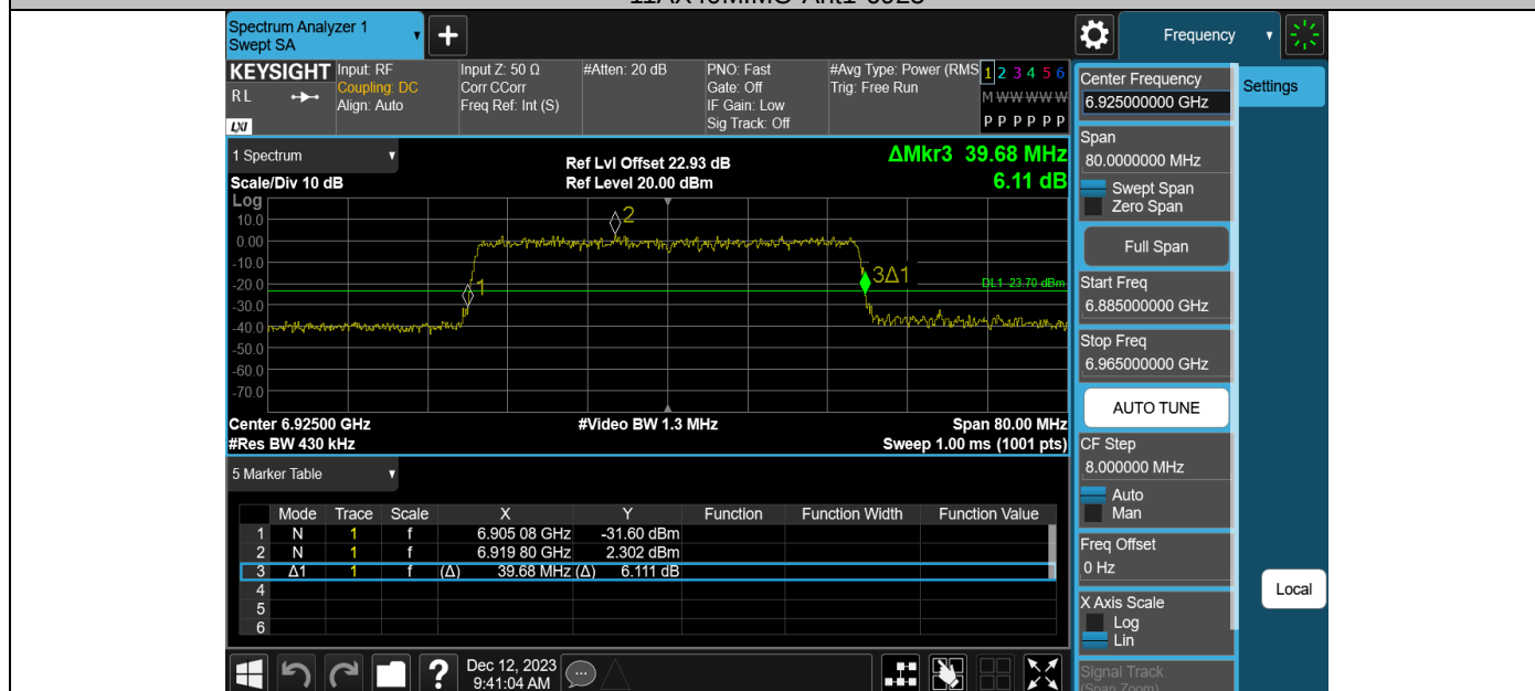
11AX40MIMO-Ant2-6925
