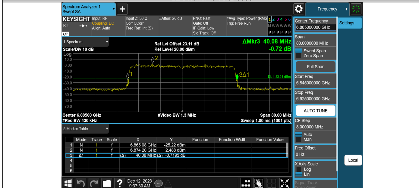
11AX40MIMO-Ant1-6925
