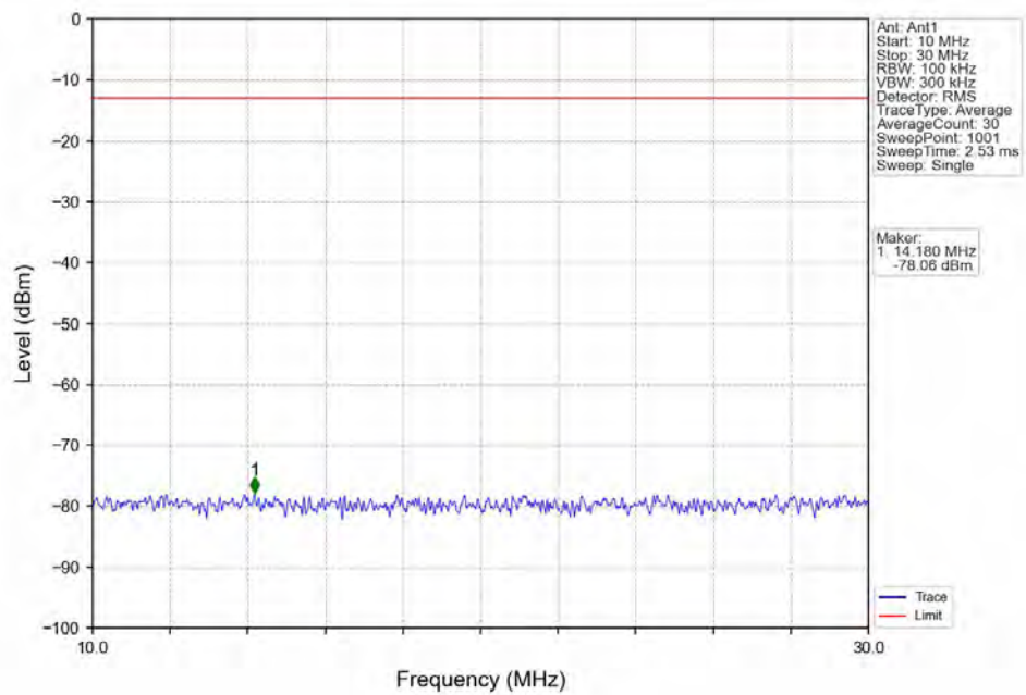
Band17_10MHz_QPSK_LCH_709MHz_RB_1_0_NTNV
