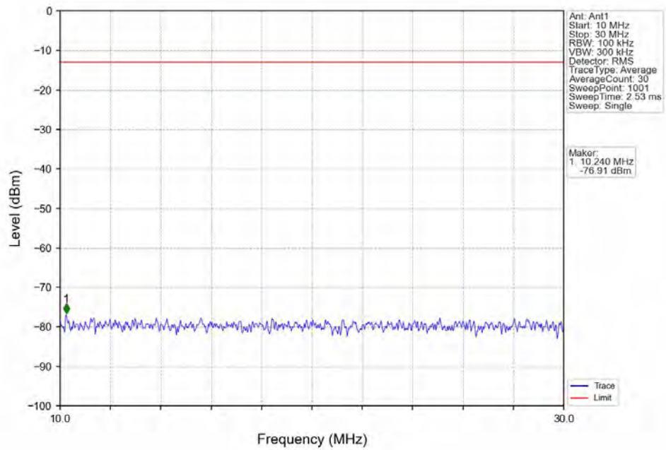
Band17_10MHz_QPSK_MCH_710MHz_RB_1_0_NTNV
