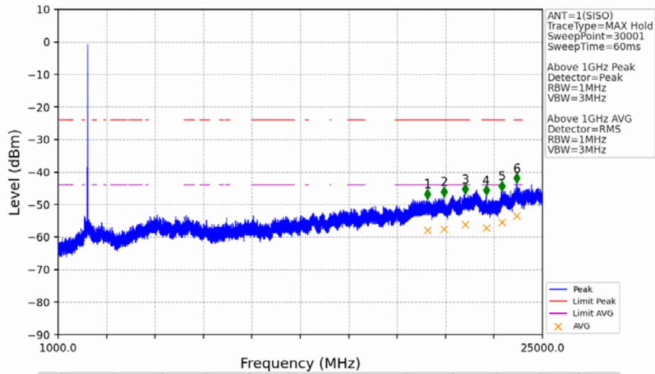
802.11b_HCH_2462MHz_Ant1 (SISO)_NTNV
