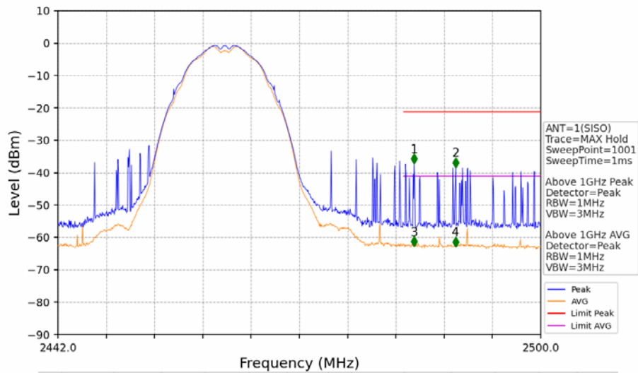
802.11b_HCH_2462MHz_Ant1 (SISO)_NTNV
