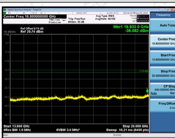
WCDMA 1900-LCH
