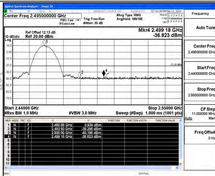
11G_Ant_Low_2412_AV
