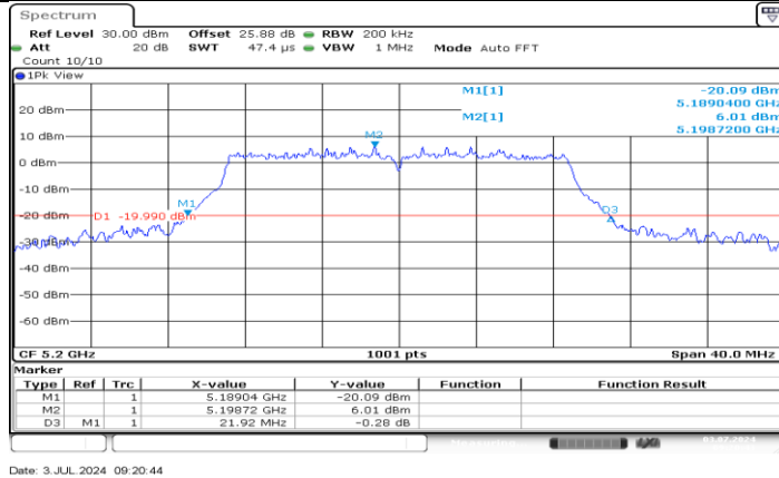
11N20SISO_Ant1_5200
