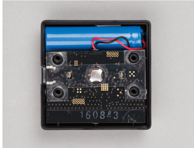
PCB Bottom
