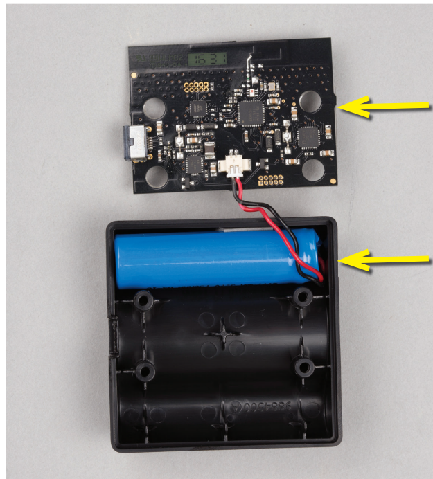
PCB Top
