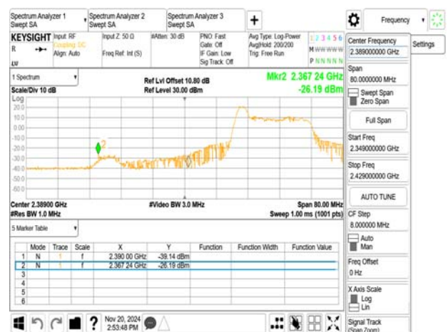
802.11ax_20MHz_2412MHz_RU26_0
