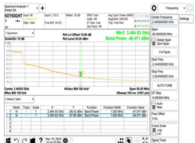
802.11n_20MHz_2442MHz
