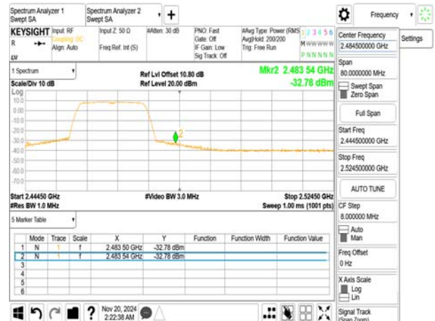
802.11n_20MHz_2472MHz
