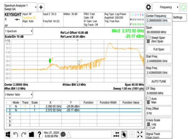
802.11ax_20MHz_2417MHz_RU52_37
