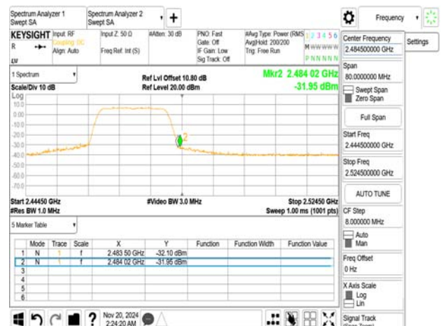
802.11n_20MHz_2472MHz
