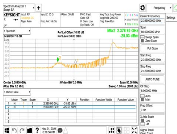
802.11ax_20MHz_2422MHz_RU52_37
