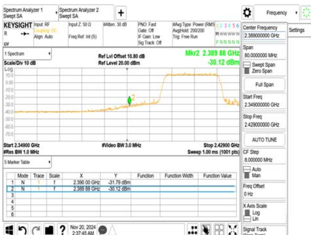
802.11ax_20MHz_2412MHz
