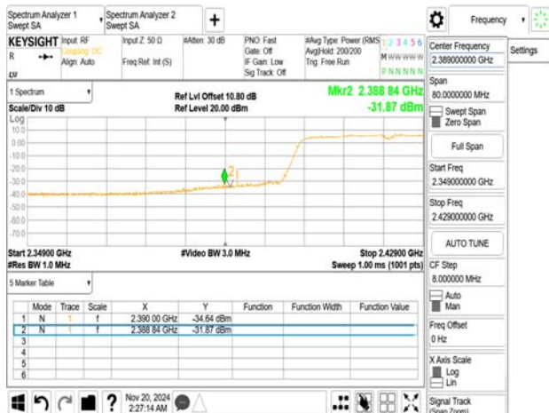
802.11n_40MHz_2427MHz
