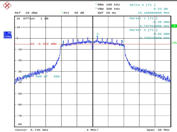
11A_Ant1_5745
