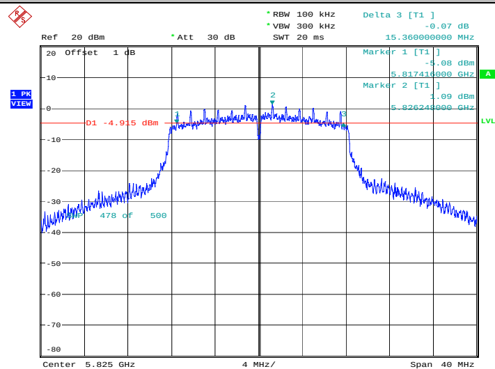
11A_Ant1_5825
