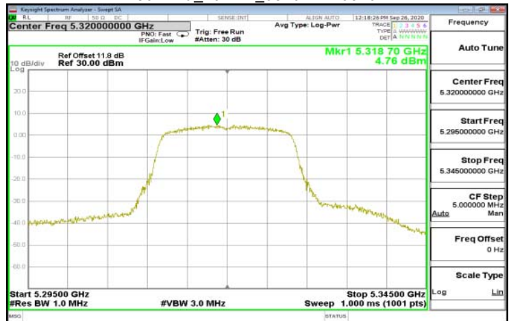
802.11a_20MHz_5320MHz-5320
