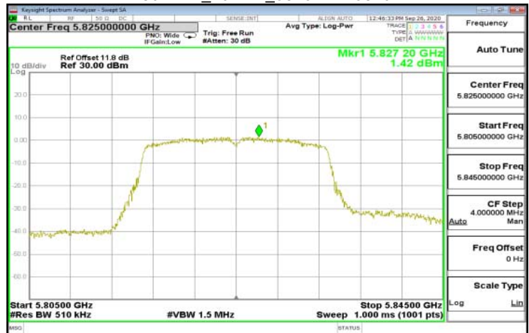
802.11n_20MHz_5825MHz-5825
