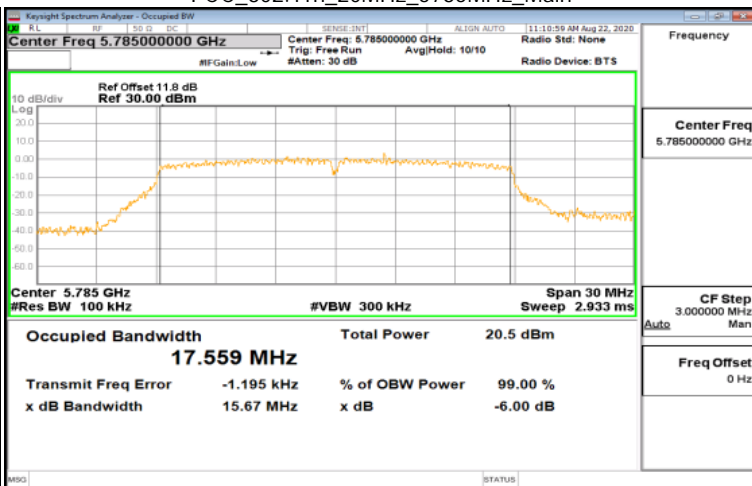
FCC_802.11n_20MHz_5785MHz_Main
