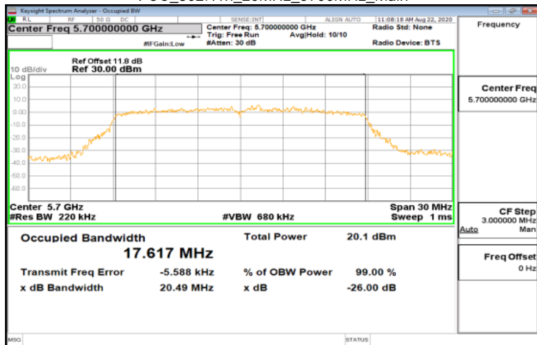
FCC_802.11n_20MHz_5700MHz_Main
