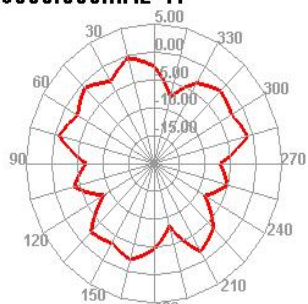
6000.000MHz H
