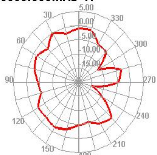
5550.000MHz H
