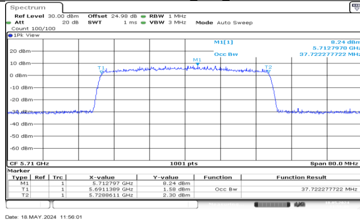
11AX40MIMO_Ant1_5710
