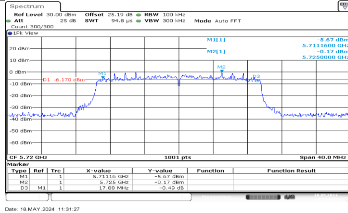
11AX20MIMO_Ant1_5720
