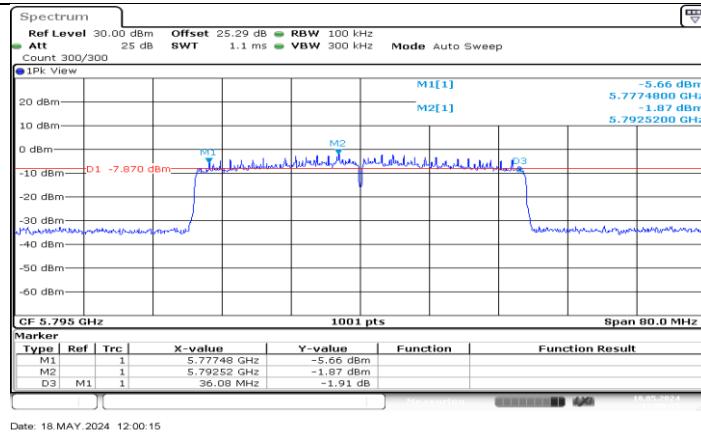
11AX40MIMO_Ant1_5795
