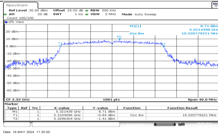
11AX20MIMO_Ant1_5320
