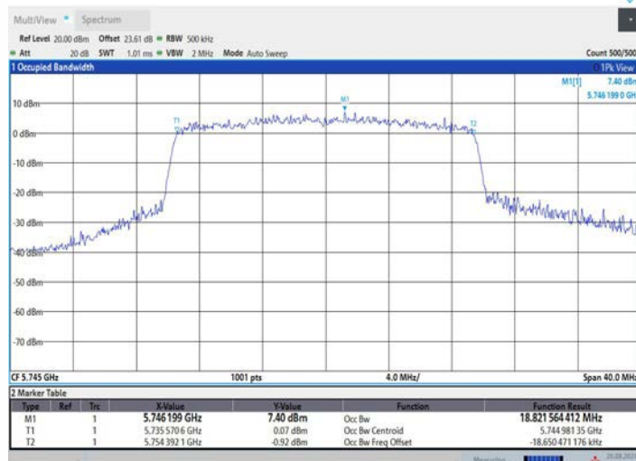
11AX20MIMO_Ant3_5745
