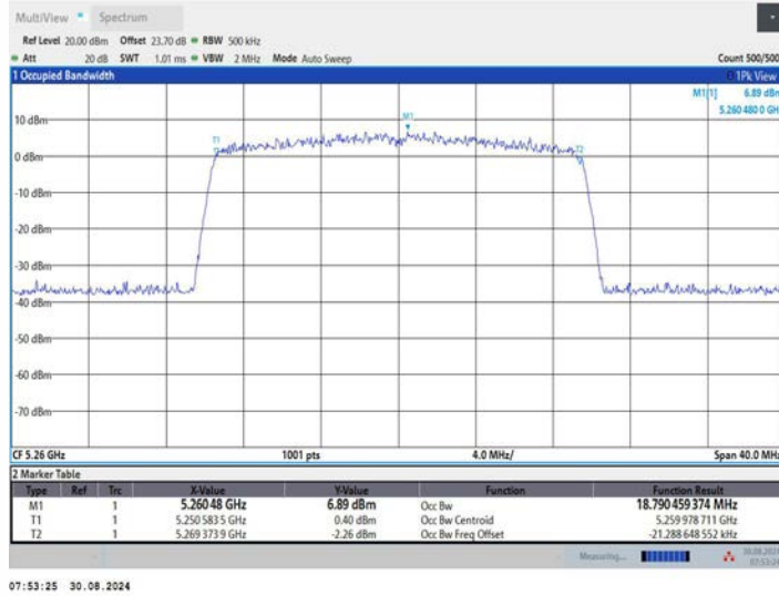
11BE20MIMO_Ant2_5260
