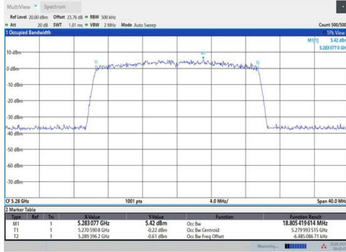
11BE20MIMO_Ant3_5280
