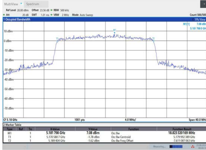
11AX20MIMO_Ant3_5180
