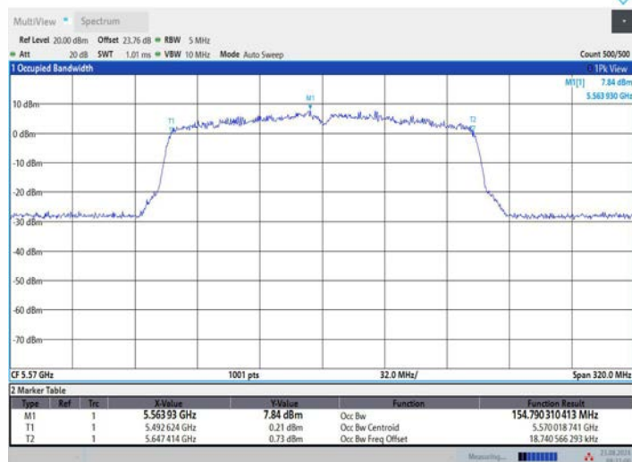
11AC160MIMO_Ant3_5570
