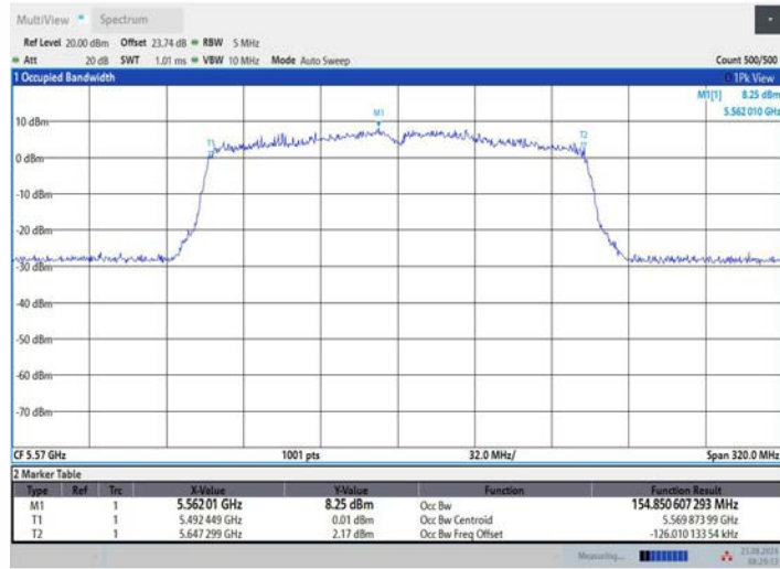
11AC160MIMO_Ant2_5570
