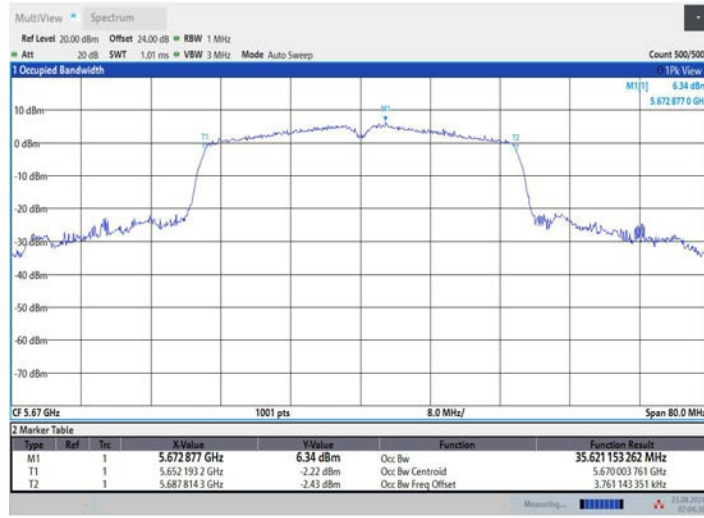
11AC40MIMO_Ant3_5670
