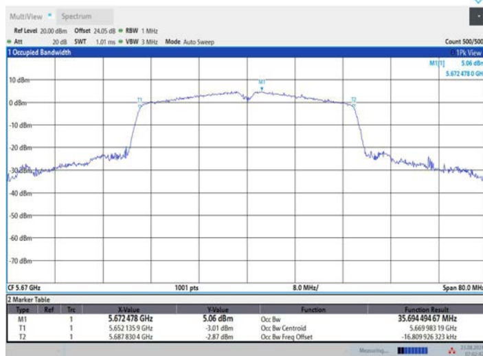
11AC40MIMO_Ant2_5670
