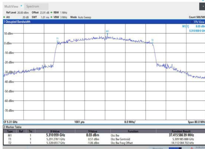
11AX40MIMO_Ant3_5310
