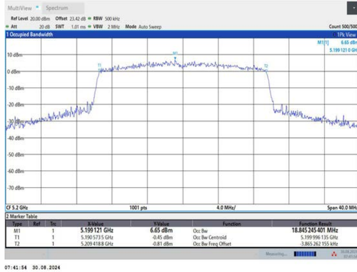
11BE20MIMO_Ant2_5200
