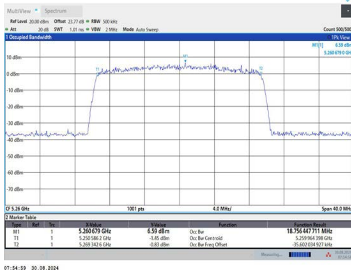
11BE20MIMO_Ant3_5260
