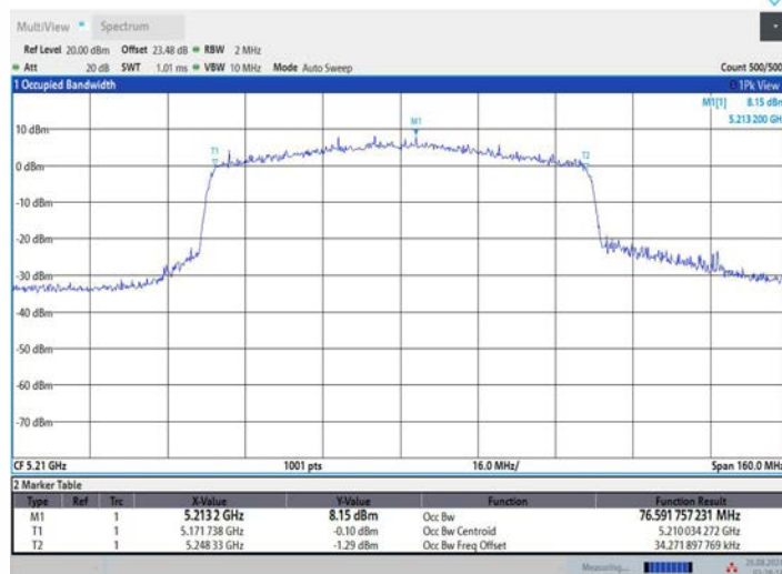
11AX80MIMO_Ant3_5210
