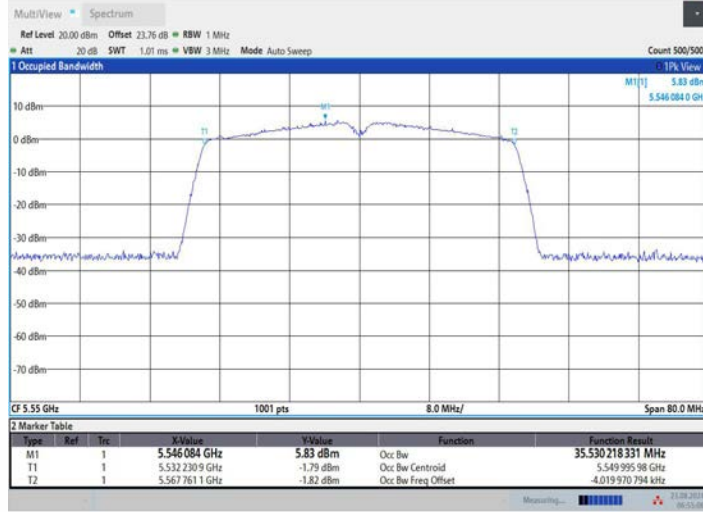
11AC40MIMO_Ant2_5550
