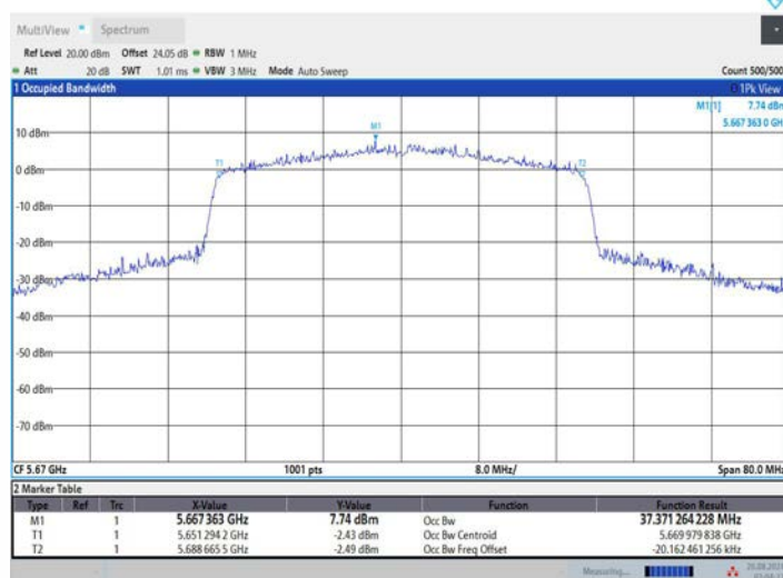
11AX40MIMO_Ant2_5670
