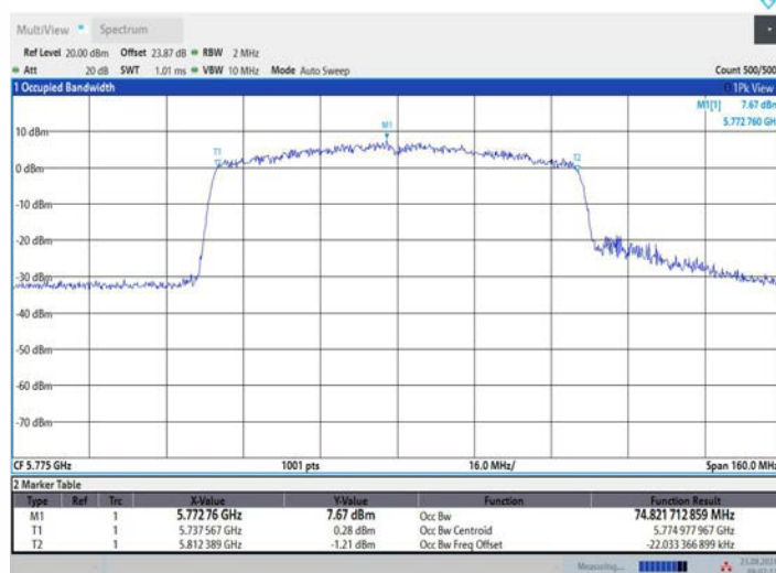
11AC80MIMO_Ant3_5775
