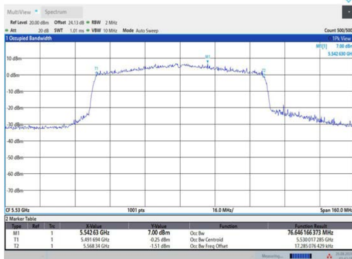
11AX80MIMO_Ant3_5530
