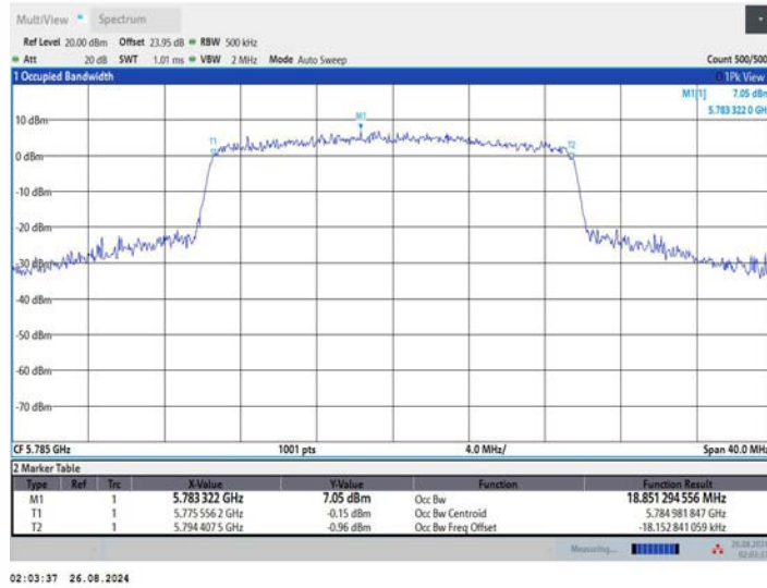
11AX20MIMO_Ant3_5785
