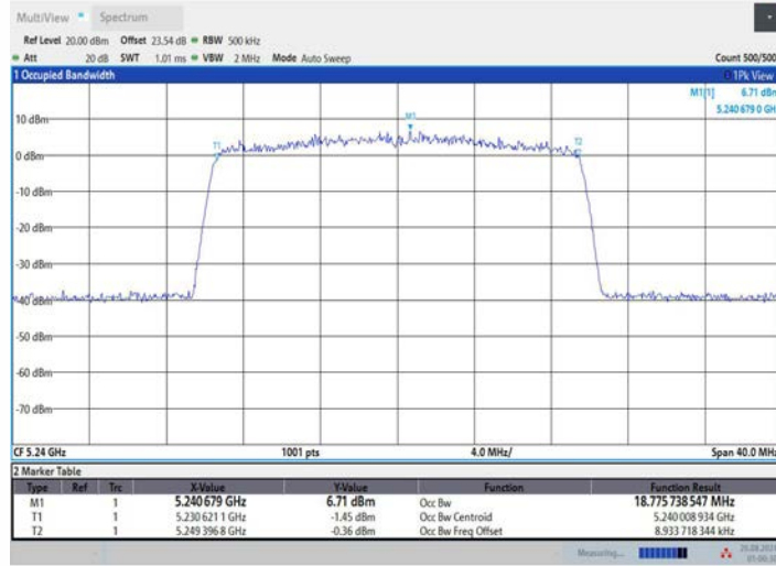
11AX20MIMO_Ant3_5240
