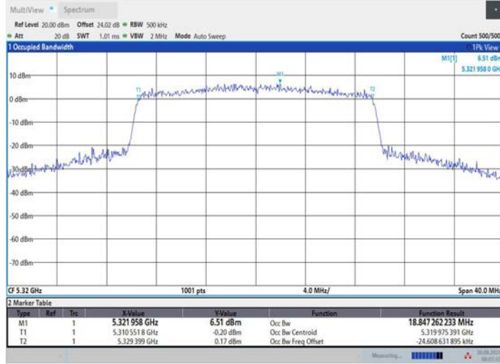
11BE20MIMO_Ant2_5320
