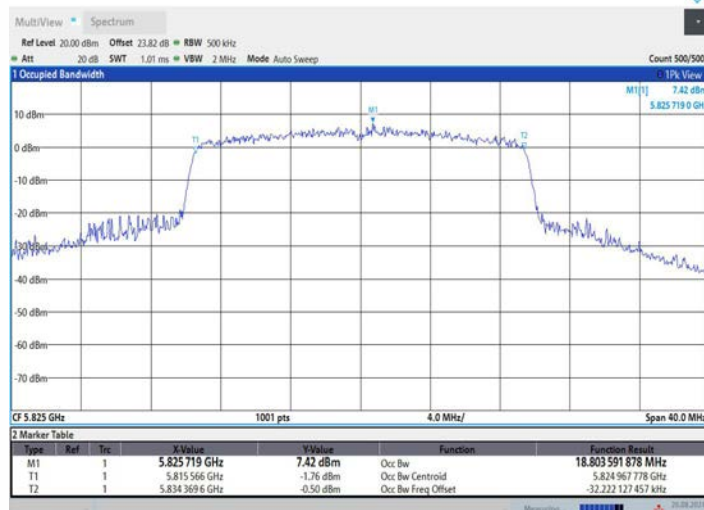
11AX20MIMO_Ant3_5825
