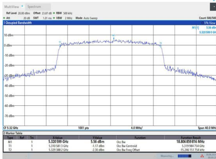
11BE20MIMO_Ant3_5320
