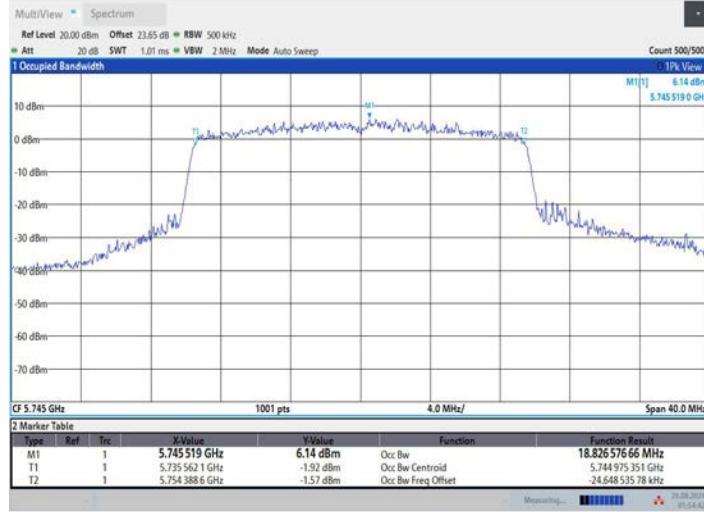
11AX20MIMO_Ant2_5745
