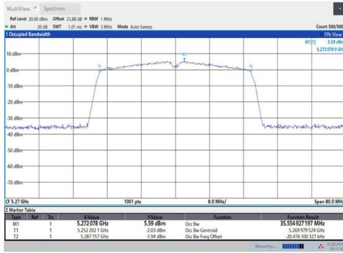
11AC40MIMO_Ant3_5270
