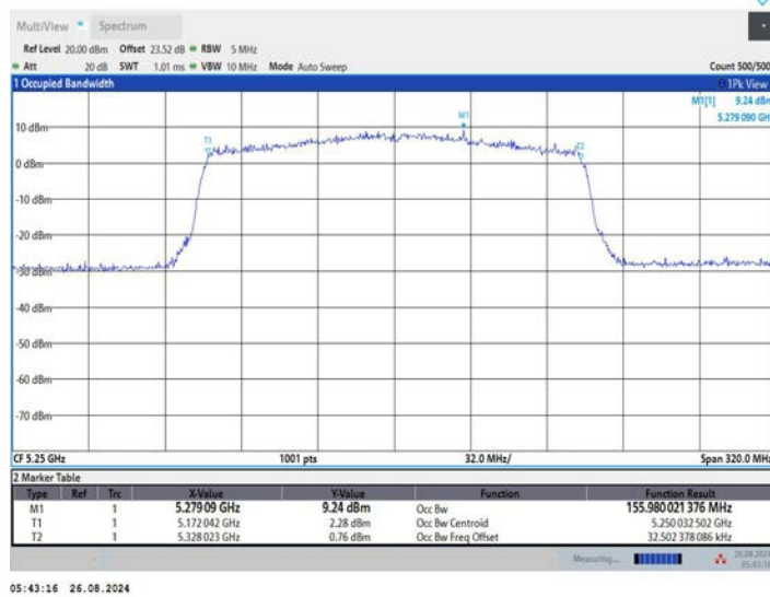
11AX160MIMO_Ant2_5250
