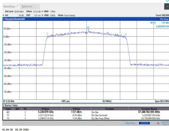
11AX40MIMO_Ant3_5230
