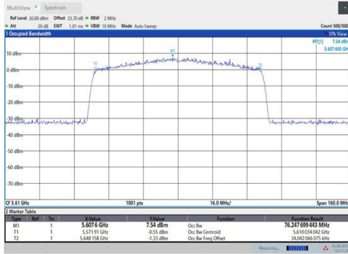
11AX80MIMO_Ant3_5610
