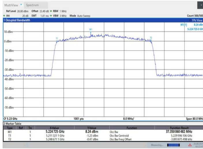
11AX40MIMO_Ant2_5230
