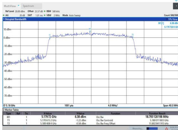
11BE20MIMO_Ant2_5180
