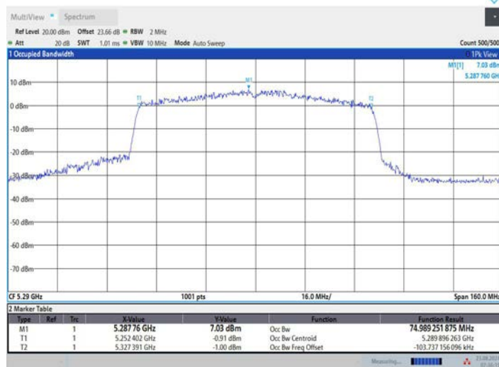
11AC80MIMO_Ant2_5290
