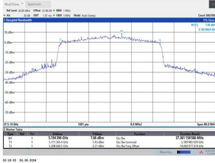
11AX40MIMO_Ant3_5190
