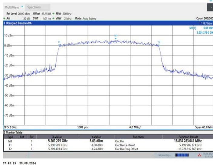
11BE20MIMO_Ant3_5200
