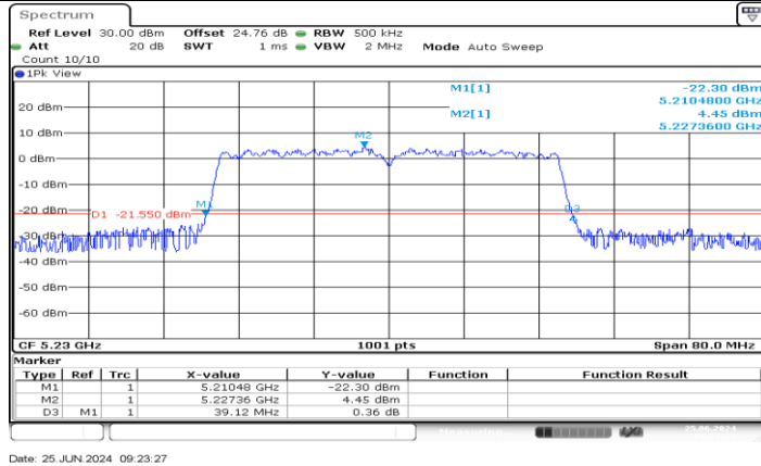
11AX40MIMO_Ant2_5230
