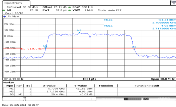
11AX20MIMO_Ant2_5720
