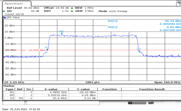
11AX80MIMO_Ant1_5530
