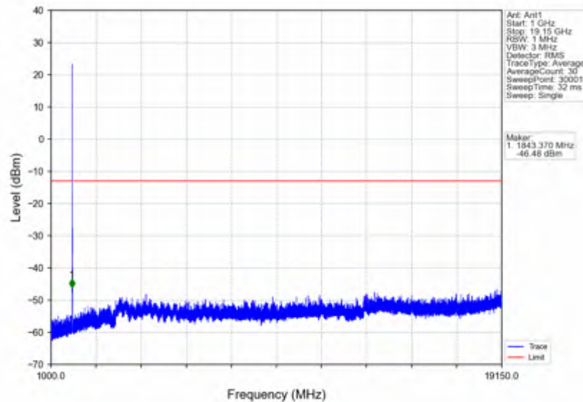
n25_15kHz_SISO_NTNV_10MHz_DFT-s-OFDM QPSK_1855MHz_Inner_1RB_Left
