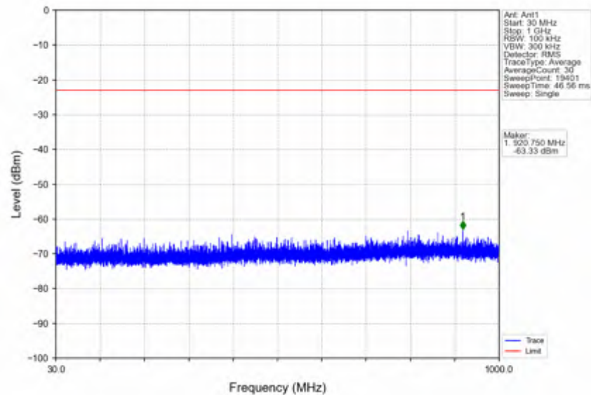
n25_15kHz_SISO_NTNV_10MHz_DFT-s-OFDM QPSK_1855MHz_Inner_1RB_Left
