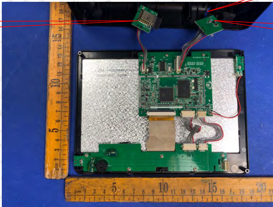
915MHz Module
