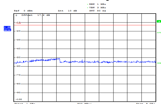
WCDMA Band V CH-High 1GHz ~ 9GHz
