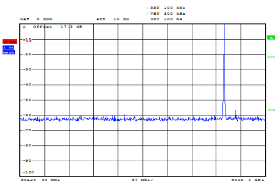
GSM 850 CH-Middle 30MHz ~ 1GHz
