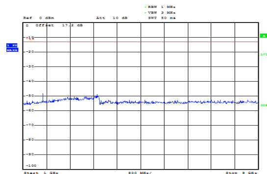
WCDMA Band V CH-Middle 1GHz ~ 9GHz
