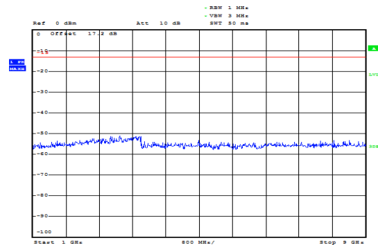
WCDMA Band V CH-Low 1GHz ~ 9GHz
