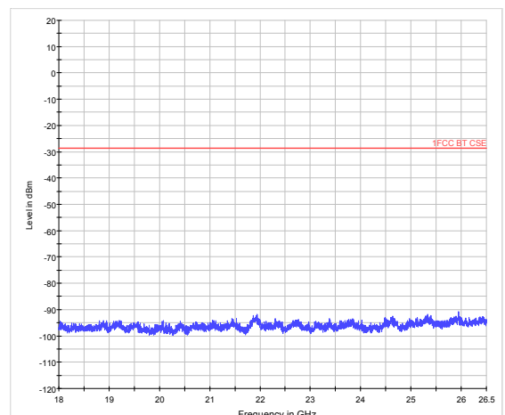
BLE CH39 18GHz to 26.5GHz
