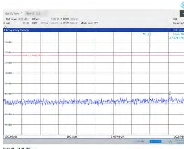
Band42-20MHz-QPSK-42190-1RB#0-Range2:0.15~30MHz
