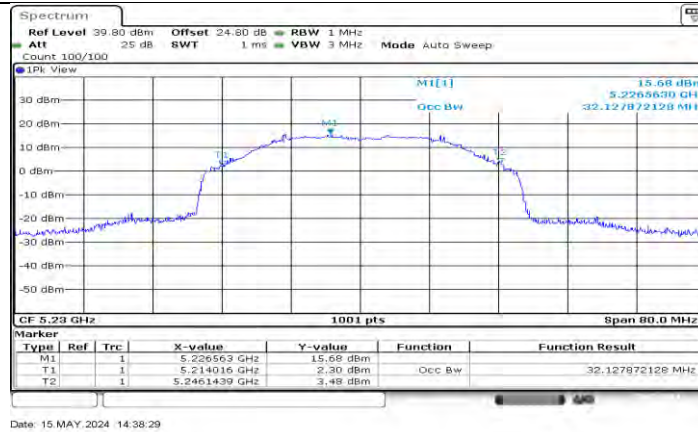
SRD 40M Ant0 5230
