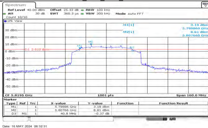
SRD 60M Ant0 5819.5
