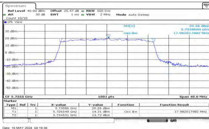
SRD 20M Ant0 5735.5
