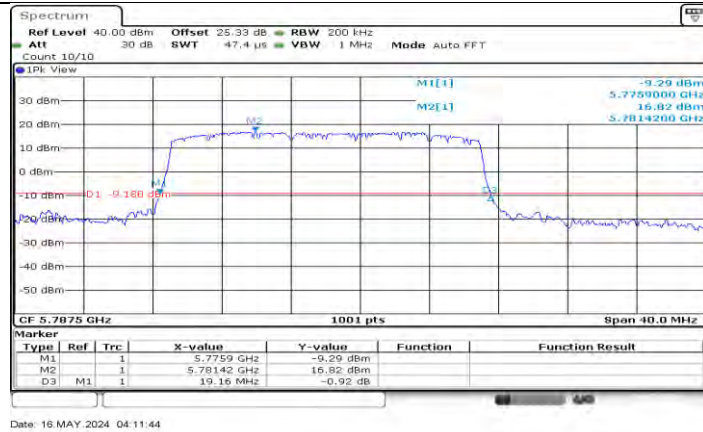
SRD 20M Ant1 5787.5
