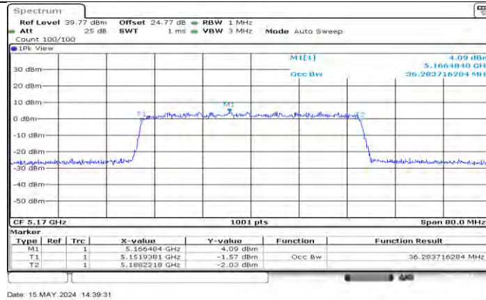
SRD 40M Ant0 5170
