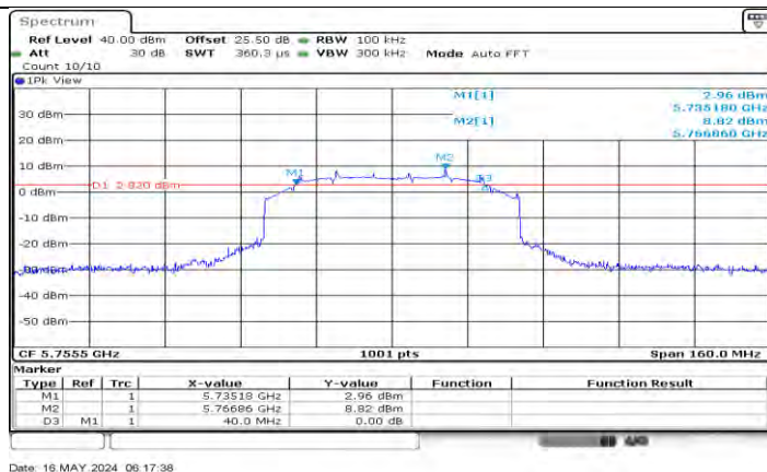
SRD 60M Ant0 5755.5
