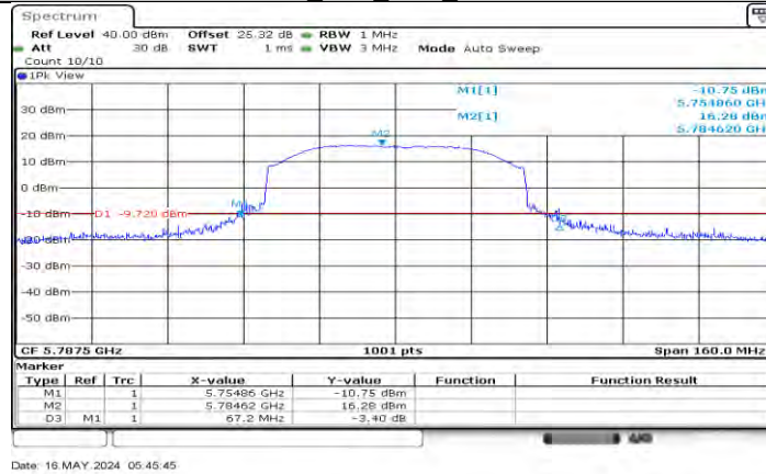
SRD 60M Ant0 5787.5
