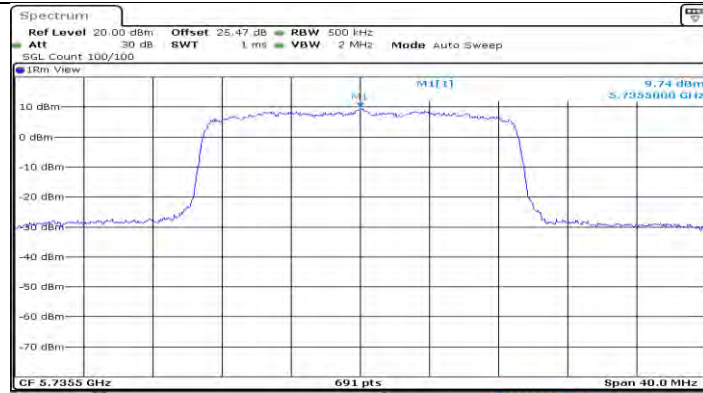
SRD 20M Ant0 5735.5
