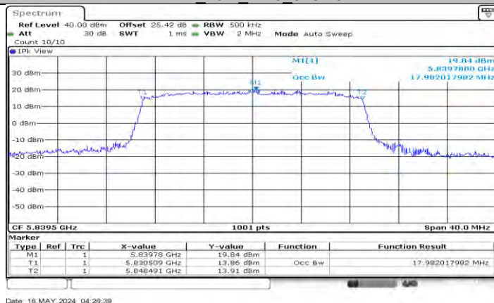
SRD 20M Ant0 5839.5
