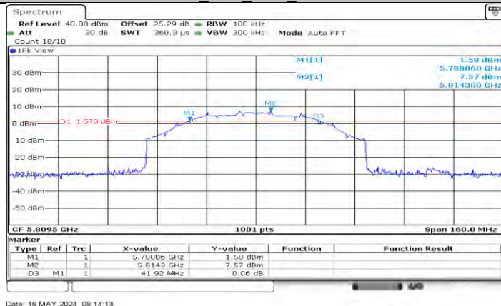
SRD 80M Ant0 5809.5
