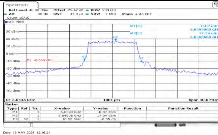
SRD 10M Ant0 5844.5
