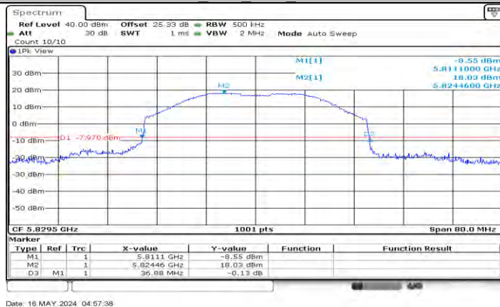
SRD 40M Ant0 5829.5
