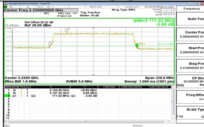
11AX160MIMO_Ant3_5250
