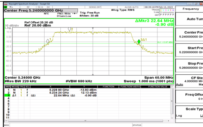
11BE20MIMO_Ant3_5240
