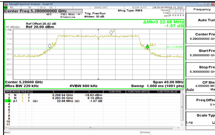
11BE20MIMO_Ant1_5280
