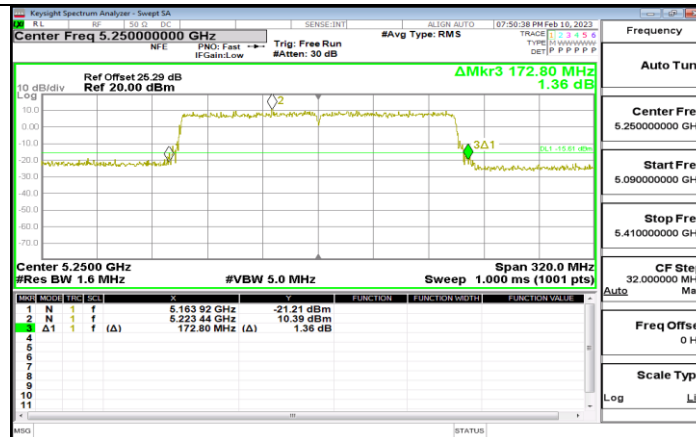
11AX160MIMO_Ant1_5250
