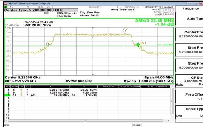
11BE20MIMO_Ant3_5280
