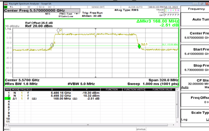
11AX160MIMO_Ant1_5570
