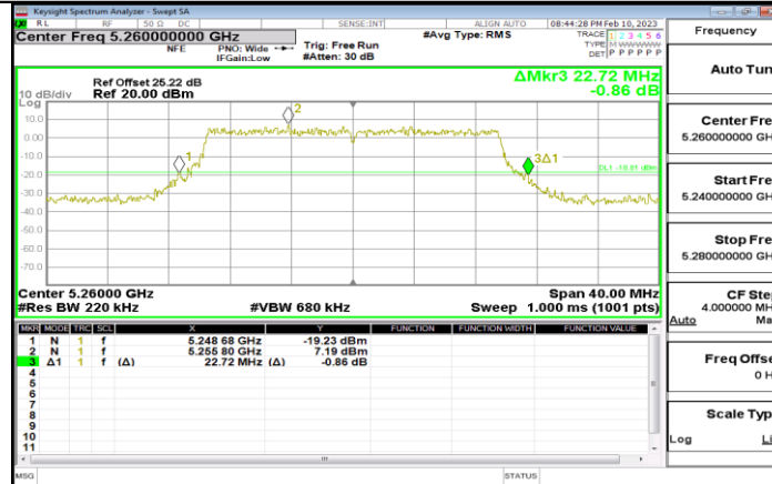
11BE20MIMO_Ant3_5260
