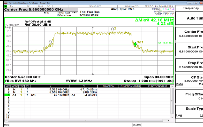
11AX40MIMO_Ant1_5550
