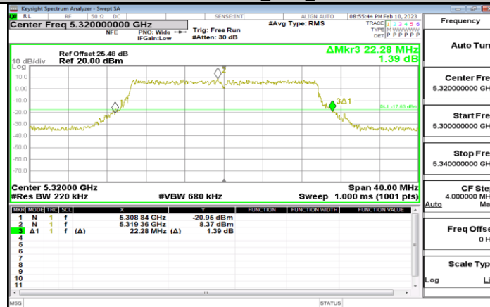
11BE20MIMO_Ant1_5320
