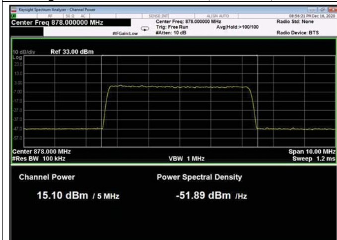
Figure 136: QPSK 5MHz B.W.; 878.0MHz, 15kHz
