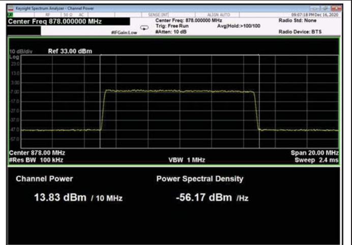
Figure 143: QPSK 10MHz B.W.; 878.0MHz, 15kHz
