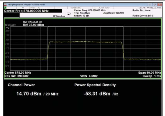
Figure 119: 256QAM 20MHz B.W.; 878.0MHz, 15kHz
