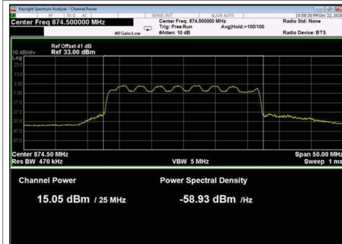
Figure 42: 16QAM 25MHz B.W.; 874.5MHz, 30kHz
