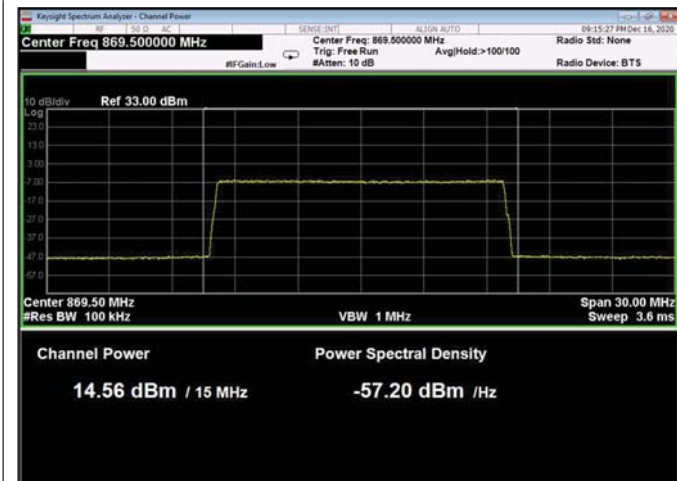
Figure 150: QPSK 15MHz B.W.; 869.5MHz, 30kHz
