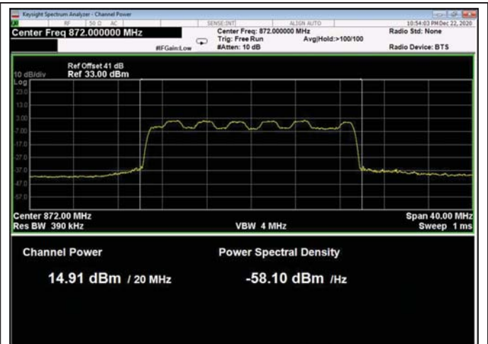
Figure 33: 16QAM 20MHz B.W.; 872.0MHz, 30kHz
