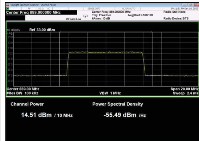
Figure 148: QPSK 10MHz B.W.; 889.0MHz, 60kHz
