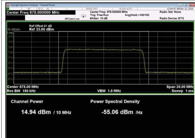
Figure 102: 256QAM 10MHz B.W.; 878.0MHz, 30kHz
