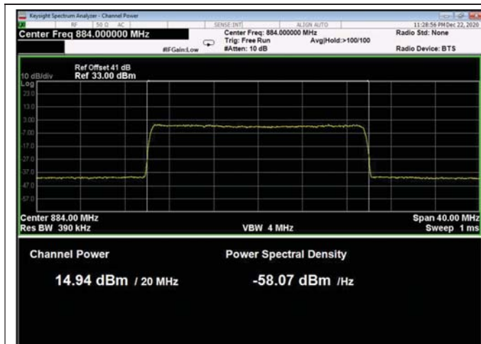
Figure 80: 64QAM 20MHz B.W.; 884.0MHz, 15kHz
