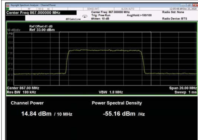
Figure 100: 256QAM 10MHz B.W.; 867.0MHz, 60kHz
