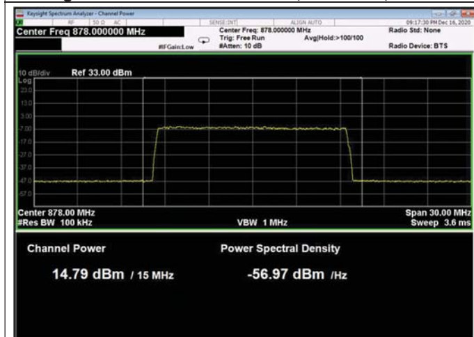
Figure 154: QPSK 15MHz B.W.; 878.0MHz, 60kHz
