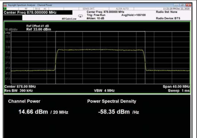
Figure 77: 64QAM 20MHz B.W.; 878.0MHz, 15kHz
