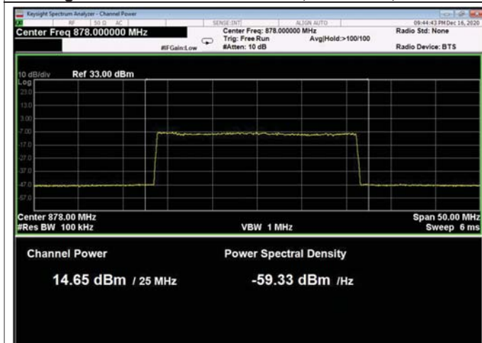
Figure 172: QPSK 25MHz B.W.; 878.0MHz, 60kHz
