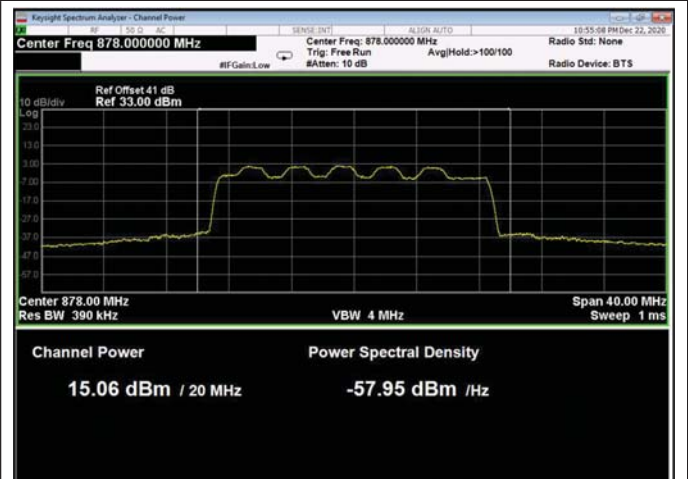
Figure 37: 16QAM 20MHz B.W.; 878.0MHz, 60kHz
