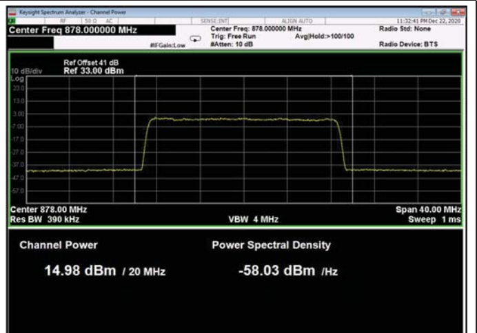
Figure 79: 64QAM 20MHz B.W.; 878.0MHz, 60kHz
