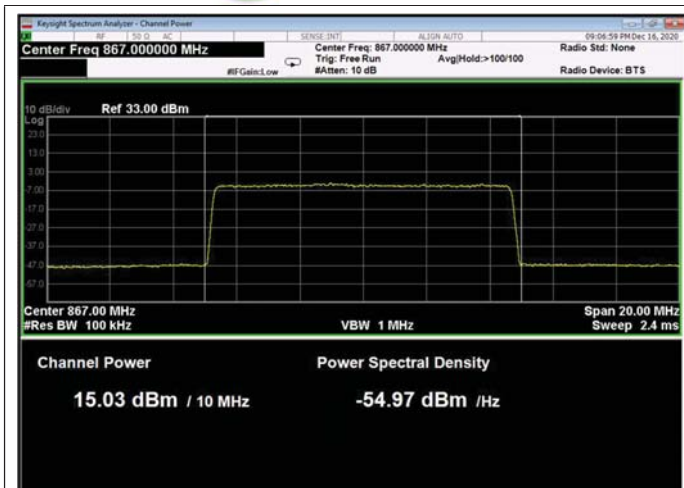
Figure 140: QPSK 10MHz B.W.; 867.0MHz, 15kHz
