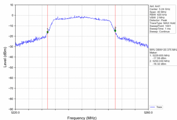
802.11ac (20MHz)
