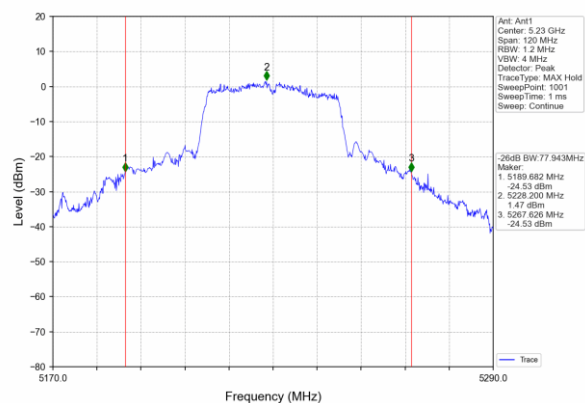
802.11ac (40MHz)
