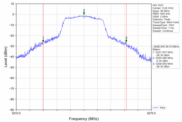
802.11ac (20MHz)
