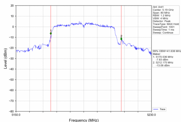
802.11ac (40MHz)
