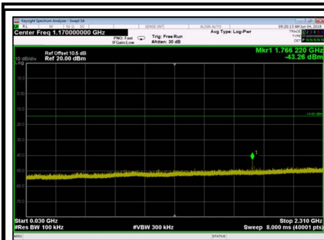
,Plot 3,30MHz~2310MHz-802.11b,2462MHz
