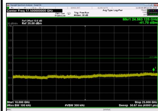
,Plot 5,10000MHz~25000MHz-802.11n(HT4 0) ,2437MHz,
