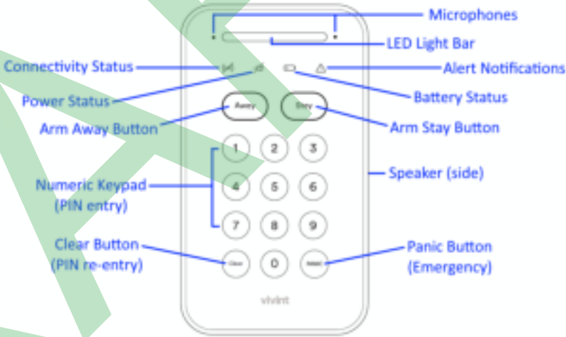
Smart Hub Lite Keypad —
