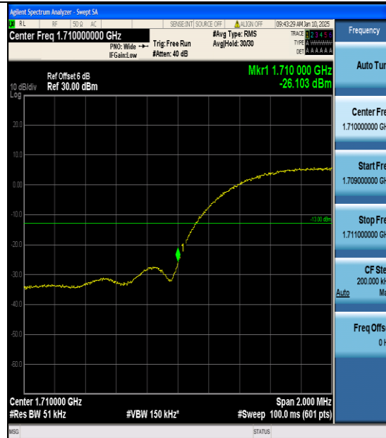
Band4-1312-1-PASS
