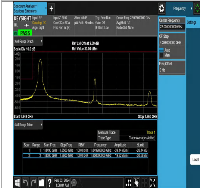
Band2_10MHz_QPSK_18650_1RB#0
