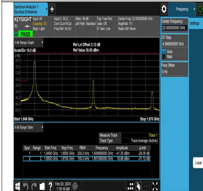
Band2_20MHz_QPSK_18700_1RB#0
