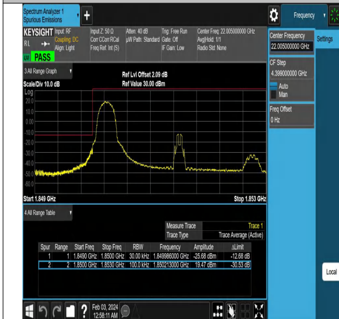
Band2_3MHz_QPSK_18615_1RB#0
