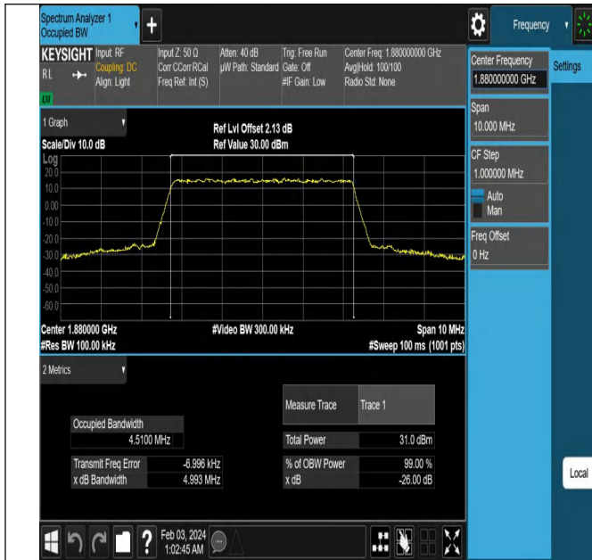
Band2-5MHz-QPSK-18900-25RB#0-PASS
