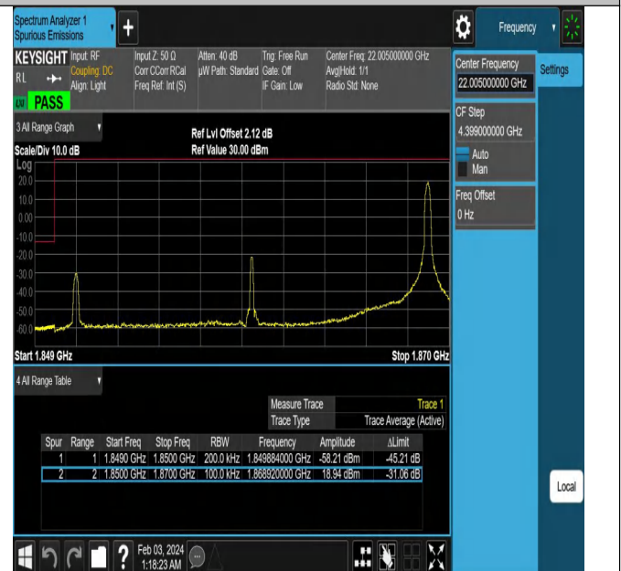
Band2_20MHz_QPSK_18700_1RB#99
