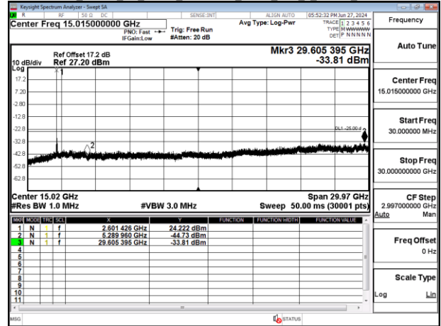
Band41_100MHz_CP_OFDM_SCS30kHz_QPSK_RB1_1_Chain0_CH509202
