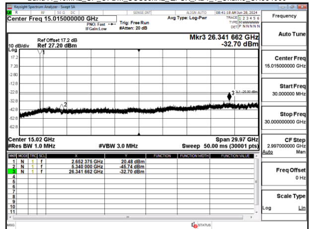
Band41 40MHz CP OFDM SCS30kHz QPSK RB1_1 Chain0 CH534000
