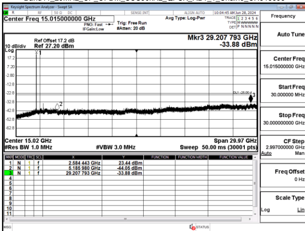
Band41 20MHz CP OFDM SCS30kHz QPSK RB1_1 Chain0 CH518598
