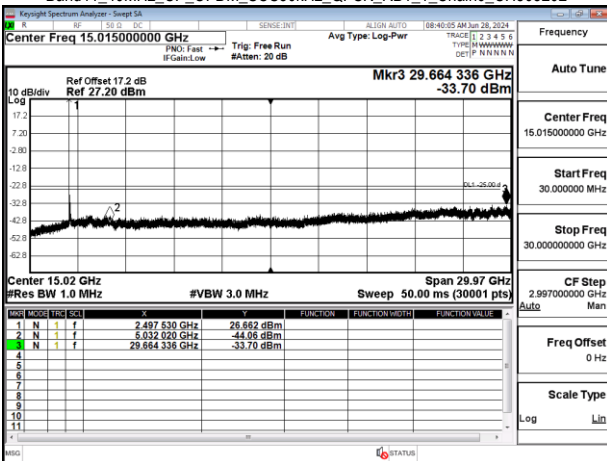
Band41 40MHz CP OFDM SCS30kHz QPSK RB1_1 Chain0 CH503202
