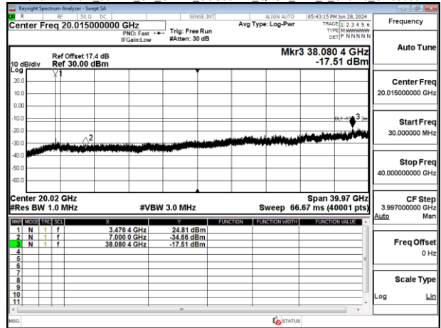
Band77-Part27_50MHz_CP_OFDM_SCS30kHz_QPSK_RB1_1_Chain0_CH635000
