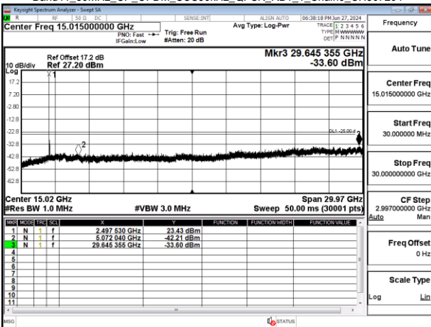
Band41 80MHz CP OFDM SCS30kHz QPSK RB1_1 Chain0 CH507204
