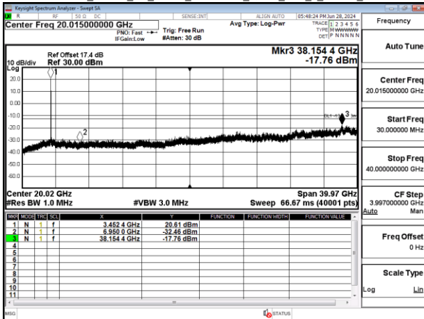
Band77-Part27_50MHz_CP_OFDM_SCS30kHz_QPSK_RB1_1_Chain0_CH631668
