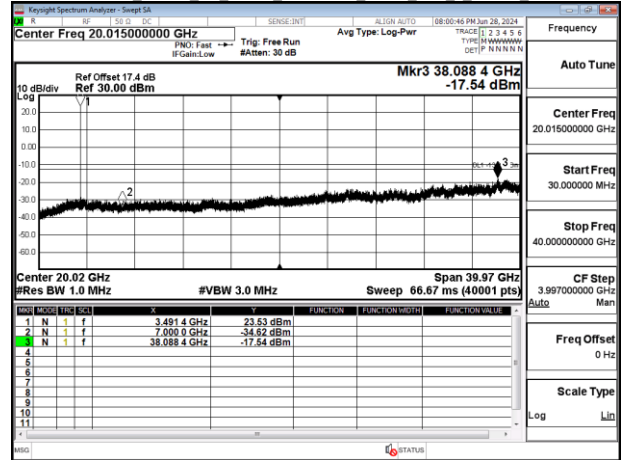
Band77-Part27 20MHz CP_OFDM_SCS30kHz_QPSK_RB1_1_Chain0_CH636000
