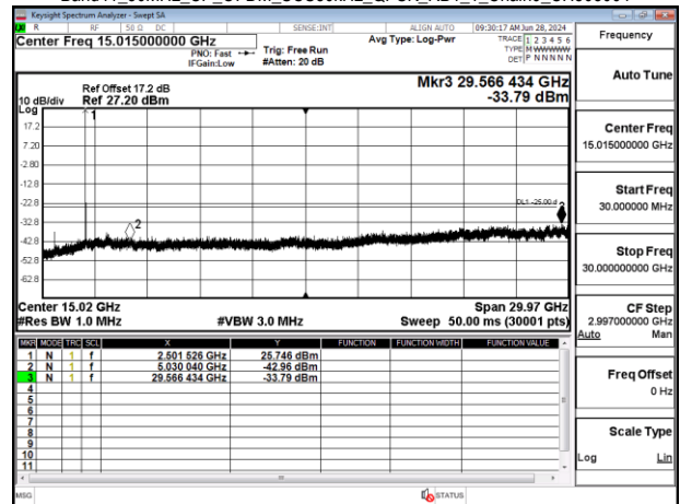
Band41 30MHz CP OFDM SCS30kHz QPSK RB1_1 Chain0 CH503004
