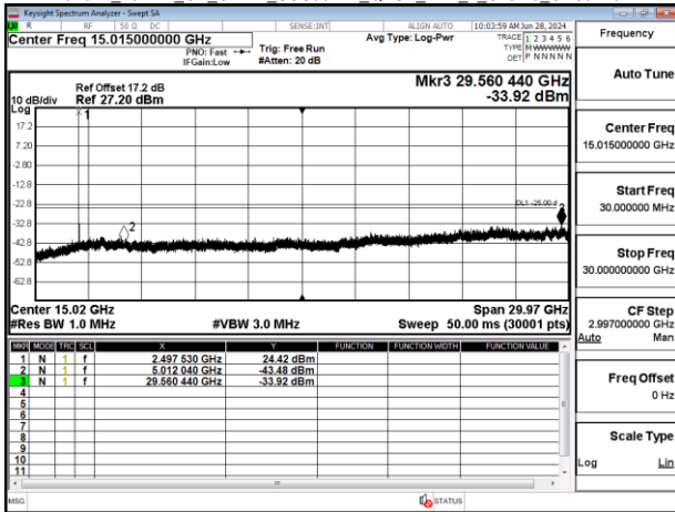
Band41 20MHz CP OFDM SCS30kHz QPSK RB1_1 Chain0 CH502002
