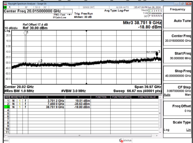
Band77-Part27_50MHz_CP_OFDM_SCS30kHz_QPSK_RB1_1_Chain0_CH648334
