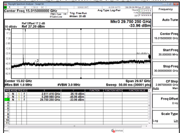
Band41 80MHz CP OFDM SCS30kHz QPSK RB1_1 Chain0 CH529998
