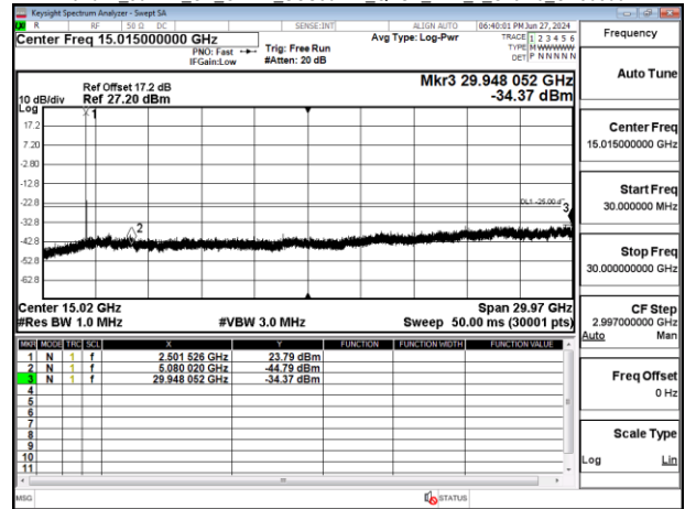
Band41 80MHz CP OFDM SCS30kHz QPSK RB1_1 Chain0 CH518598
