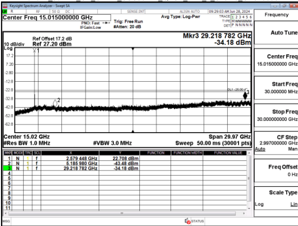
Band41 30MHz CP OFDM SCS30kHz QPSK RB1_1 Chain0 CH534996
