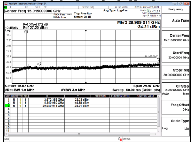
Band41 30MHz CP OFDM SCS30kHz QPSK RB1_1 Chain0 CH502200
