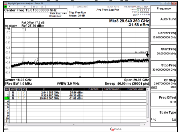
Band41_60MHz_CP_OFDM_SCS30kHz_QPSK_RB1_1_Chain0_CH505200
