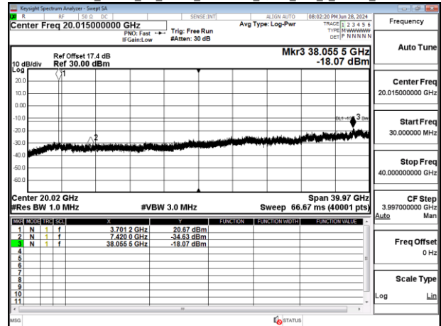
Band77-Part27 20MHz CP_OFDM_SCS30kHz_QPSK_RB1_1_Chain0_CH647334
