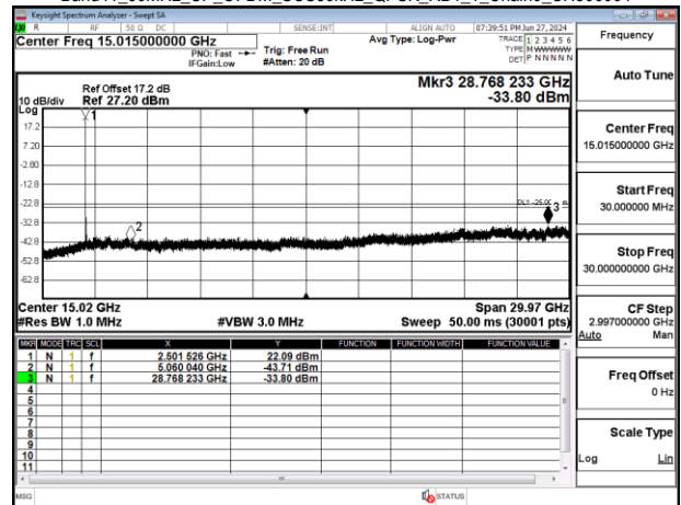
Band41_60MHz_CP_OFDM_SCS30kHz_QPSK_RB1_1_Chain0_CH506004
