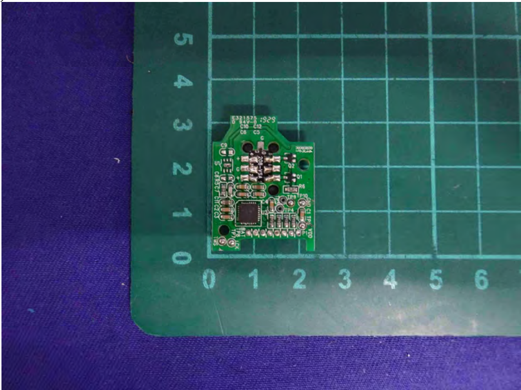
(30) EUT Photo
