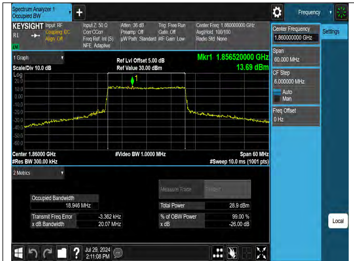
N2-20M-OBW-M-DFT-s-OFDM-Pi2 BPSK
