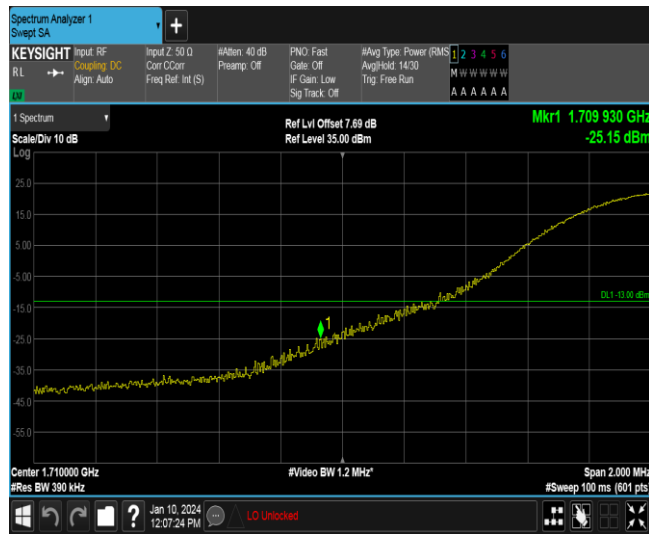
Band66-20MHz-QPSK-132072-1RB#99
