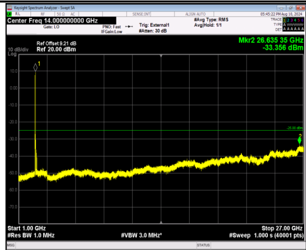
41-41-20MHz-20MHz-QPSK-QPSK-39750-39948-1RB#0-1 RB#99-1000~27000MHz-PASS
