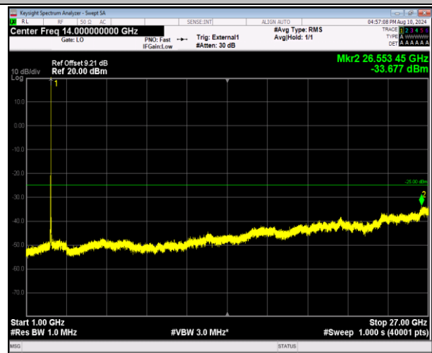
41-41-20MHz-10MHz-QPSK-QPSK-40571-40715-1RB#99- 0RB#0-1000~27000MHz-PASS
