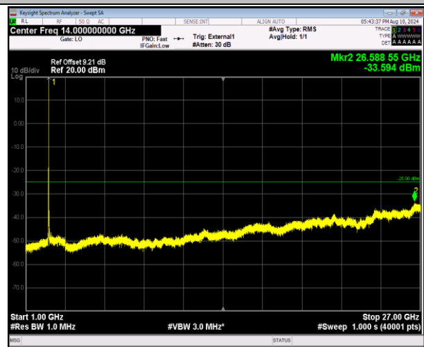
41-41-20MHz-20MHz-QPSK-QPSK-39750-39948-1RB#99- 0RB#0-1000~27000MHz-PASS
