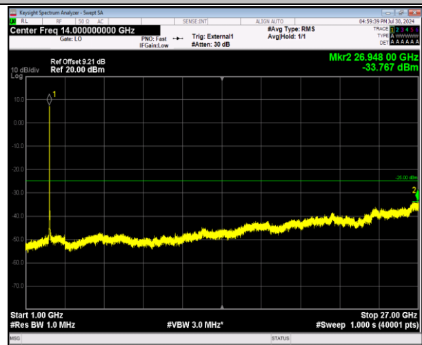
41-41-20MHz-10MHz-64QAM-64QAM-40571-40715-100RB #0-50RB#0-1000~27000MHz-PASS
