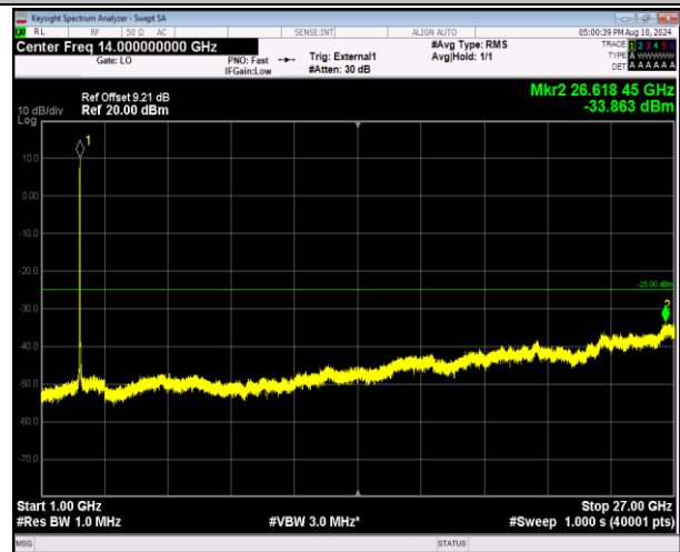
41-41-20MHz-10MHz-QPSK-QPSK-40571-40715-100RB#0 -50RB#0-1000~27000MHz-PASS
