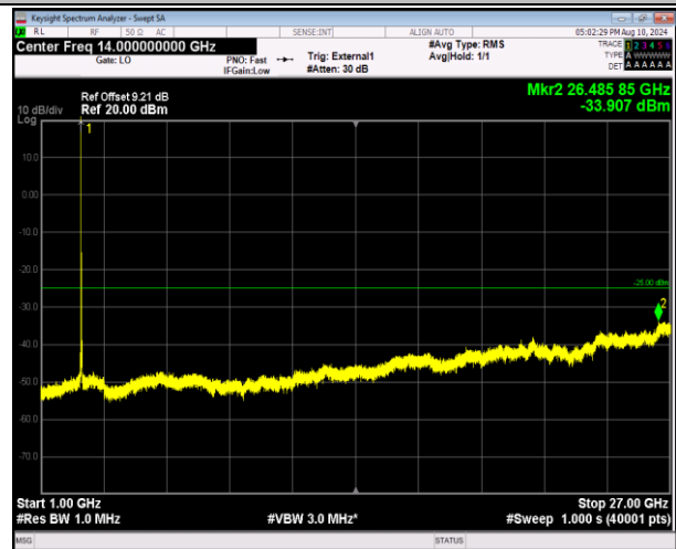
41-41-20MHz-10MHz-QPSK-QPSK-41391-41535-1RB#0-0 RB#0-1000~27000MHz-PASS
