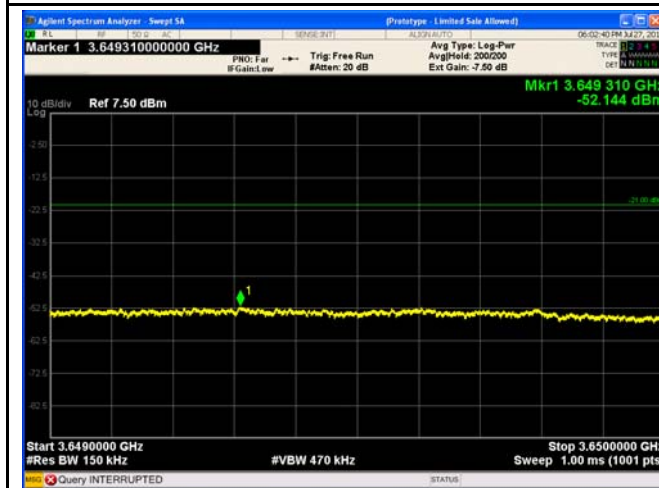
15MHz - 3649MHz-3650MHz Low CH QPSK
