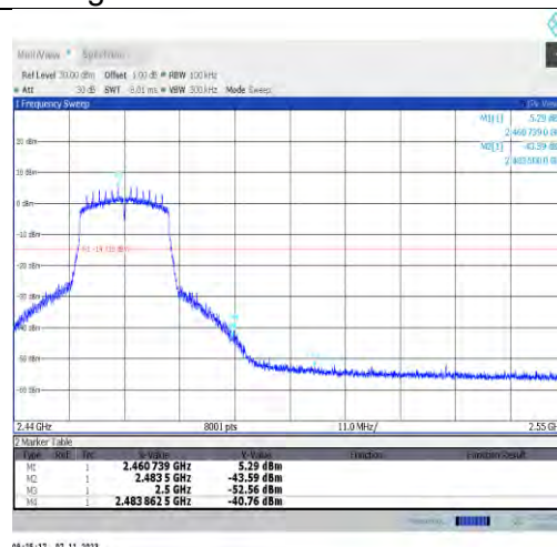
11n20ISO-Ant2-2462-PASS
