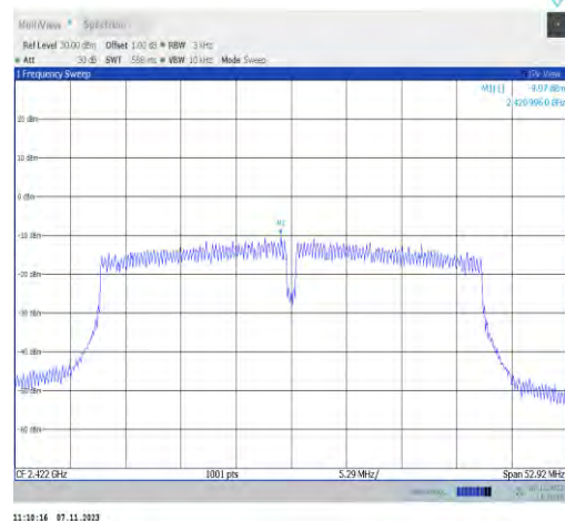
11n40ISO-Ant2-2422-PASS
