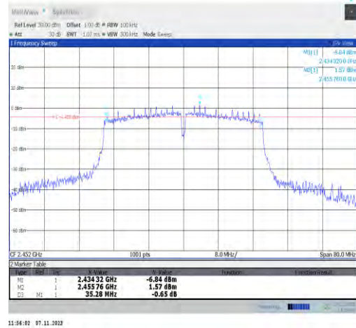
11n40ISO-Ant2-2452-PASS
