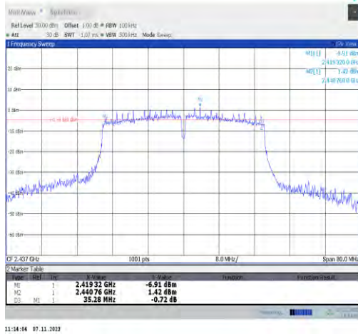
11n40ISO-Ant2-2437-PASS
