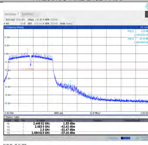
11n40ISO-Ant2-2452-PASS
