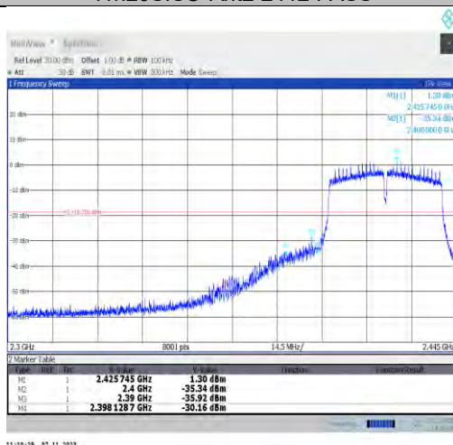
11n40ISO-Ant2-2422-PASS
