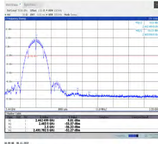
11b-Ant2-2462-PASS
