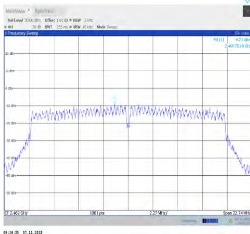
11n20ISO-Ant2-2462-PASS
