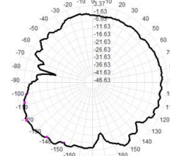
5500.0MHz Total(E2-YZ), Max= 3.37dBi
