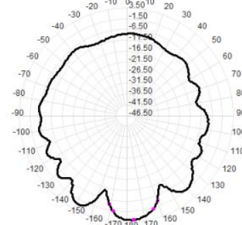
2450.0MHz Total(E1-XZ), Max= 2.08dBi
