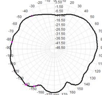
2450.0MHz Total(E2-YZ), Max= 3.50dBi
