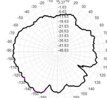
5500.0MHz Total(E1-XZ), Max= 0.75dBi
