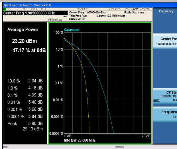
Band25-20MHz-QPSK-26590-100RB#0-PASS
