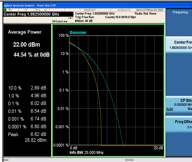
Band25-10MHz-16QAM-26365-50RB#0-PASS
