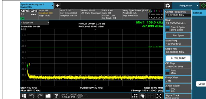
GSM850-190-5-0.15~30MHz-PASS
