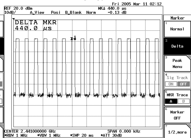
CH 39 2441MHz
