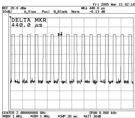
CH 78 2480MHz
