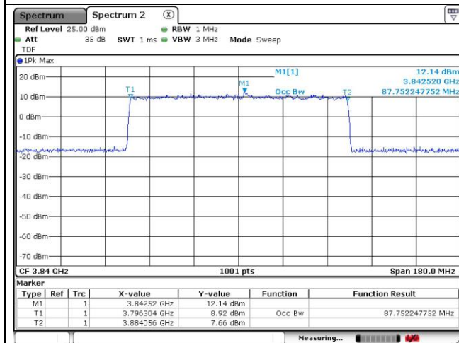
90 MHz CP-OFDM QPSK
