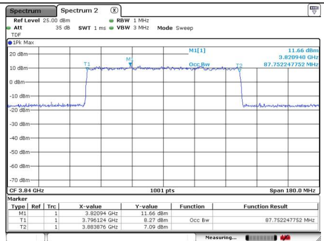
90 MHz CP-OFDM 16QAM
