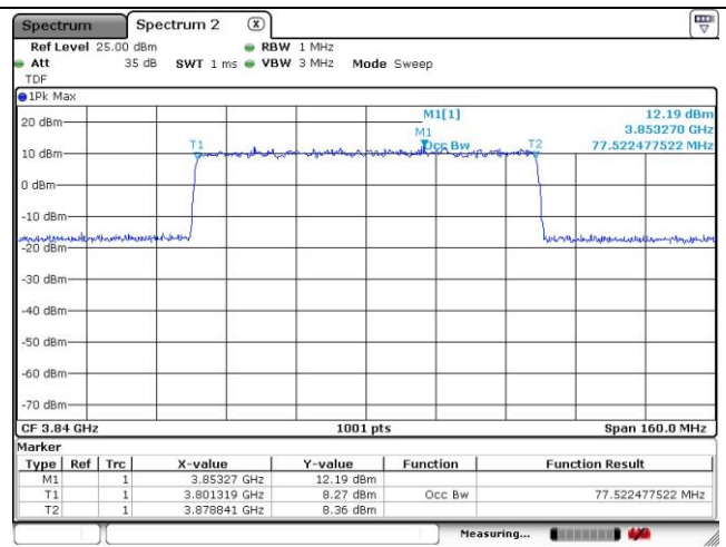
80 MHz CP-OFDM 16QAM
