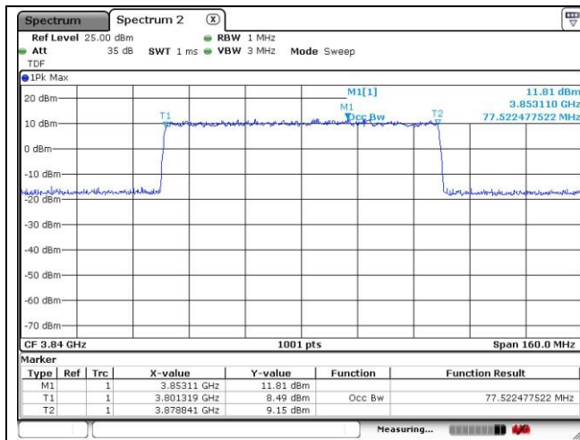
80 MHz CP-OFDM QPSK
