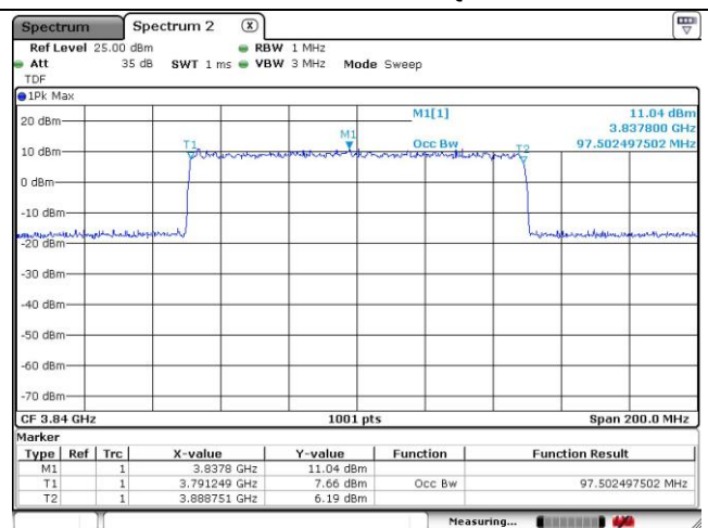
100 MHz CP-OFDM 16QAM
