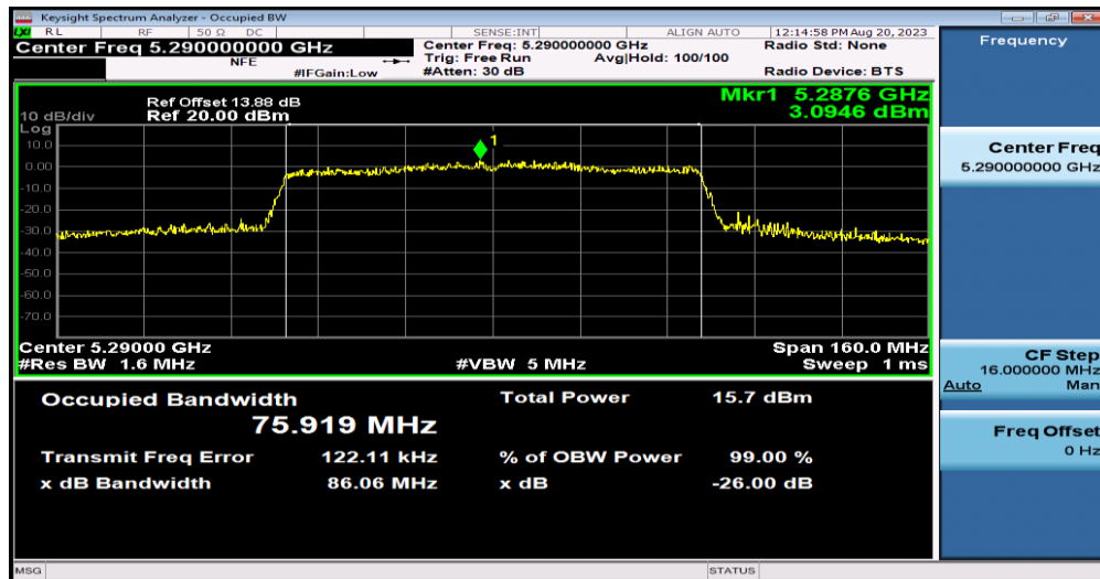
11AC80SISO-Ant1-5290
