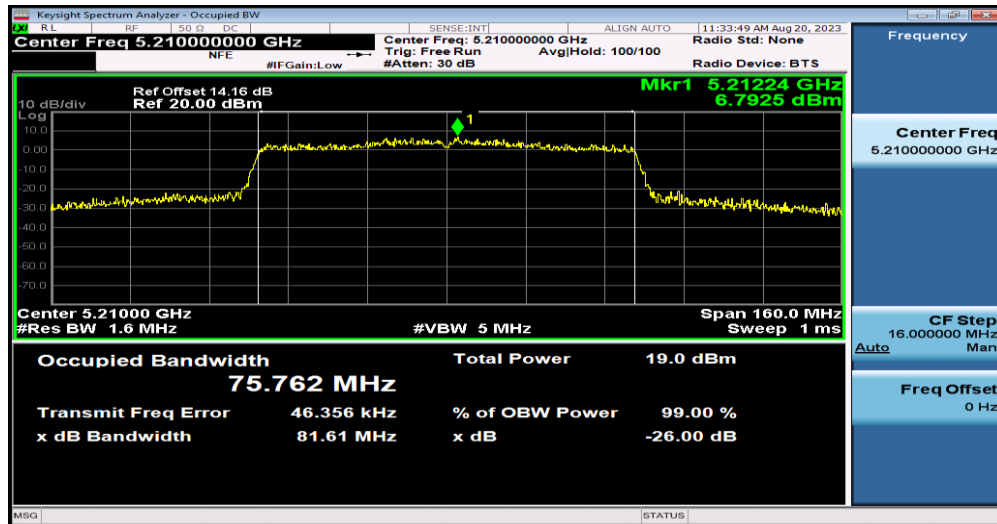
11AC80SISO-Ant1-5210
