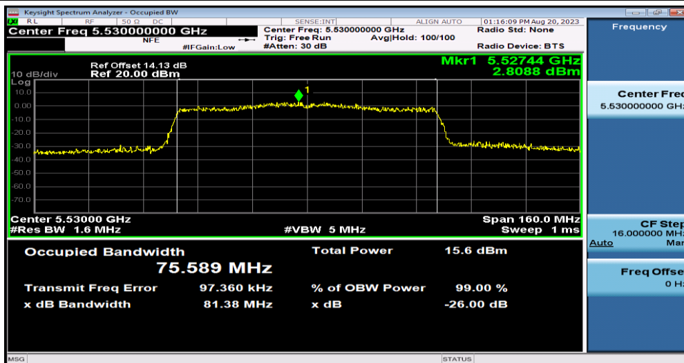
11AC80SISO-Ant1-5530
