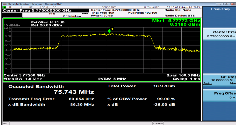
11AC80SISO-Ant1-5775
