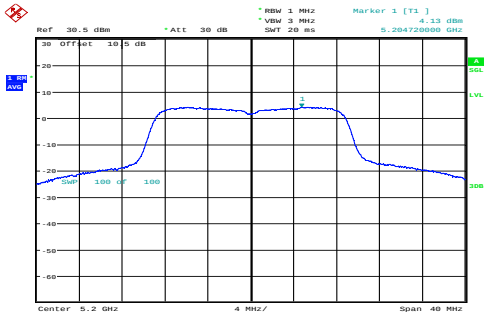
n20_5200MHz_Chain 0 4.13dBm/MHz
