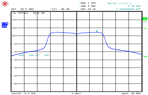
a_5200MHz_Chain 0 4.40dBm/MHz
