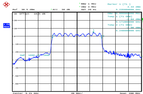
ac80_5210MHz_Chain 0 76.800MHz
