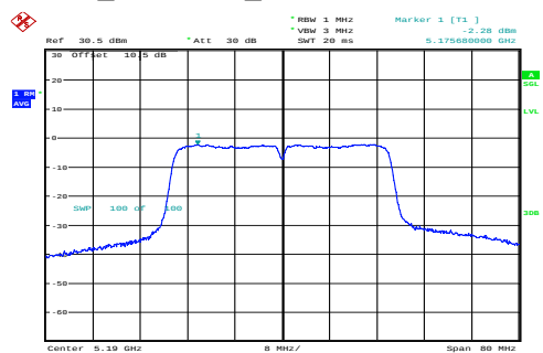
n40_5190MHz_Chain 0 -2.28dBm/MHz
