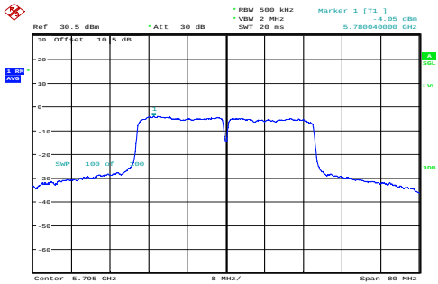
n40_5795MHz_Chain 0 -4.05dBm/MHz
