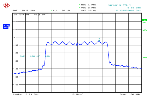
ac80_5210MHz_Chain 0 -5.10dBm/MHz
