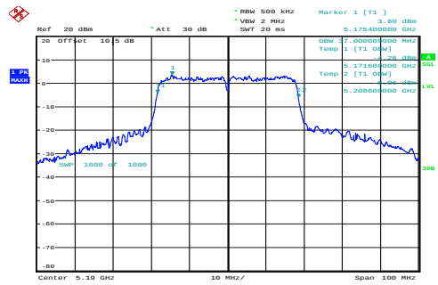
n40_5190MHz_Chain 0 37.000MHz
