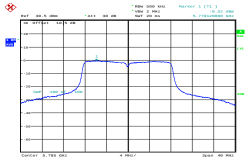
a_5785MHz_Chain 0 -0.52dBm/MHz
