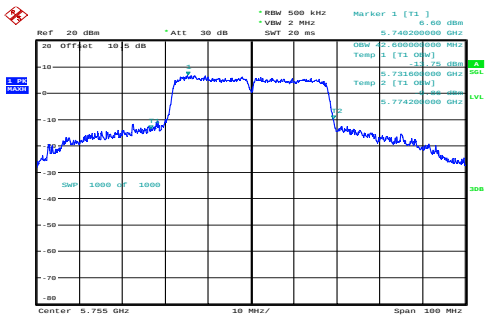
n40_5755MHz_Chain 0 42.600MHz
