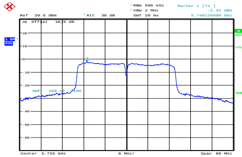
n40_5755MHz_Chain 0 -2.42dBm/MHz
