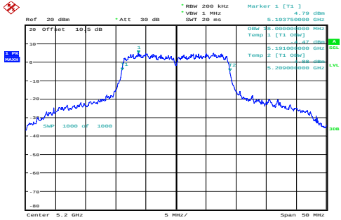
n20_5200MHz_Chain 0 18MHz
