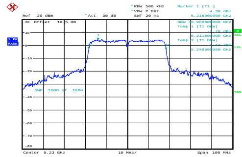
n40_5230MHz_Chain 0 36.900MHz
