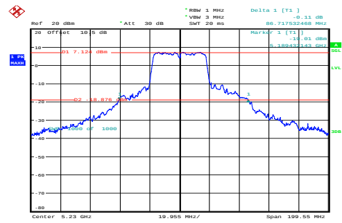
n40_5230MHz_Chain 0 86.718MHz
