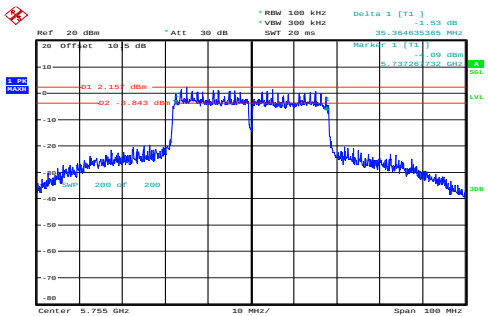
n40_5755MHz_Chain 0 35.365MHz
