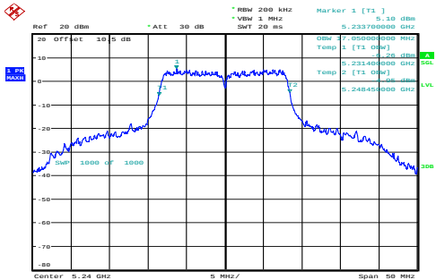
a_5240MHz_Chain 0 17.050MHz
