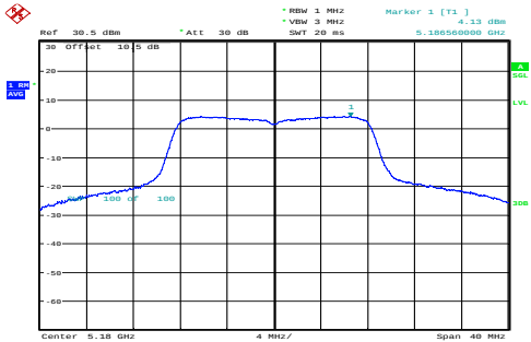
a_5180MHz_Chain 0 4.13dBm/MHz
