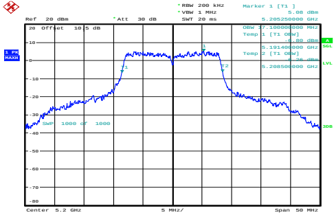
a_5200MHz_Chain 0 17.100MHz
