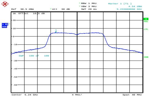
a_5240MHz_Chain 0 4.54dBm/MHz
