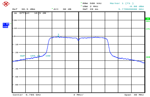
n20_5785MHz_Chain 0 -0.88dBm/MHz
