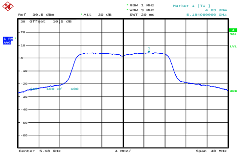
n20_5180MHz_Chain 0 4.03dBm/MHz
