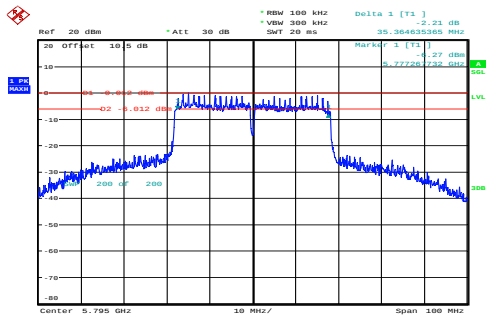
n40_5795MHz_Chain 0 35.365MHz
