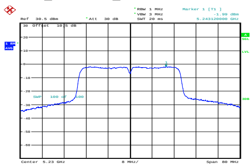
n40_5230MHz_Chain 0 -1.99dBm/MHz
