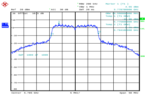
n20_5785MHz_Chain 0 18.500MHz
