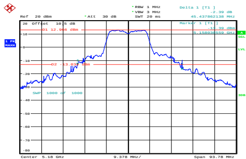
n20_5180MHz_Chain 0 45.438MHz
