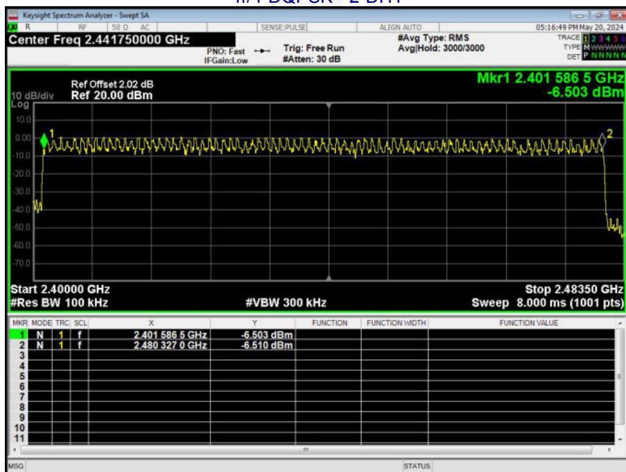
\pi/4 -DQPSK - 2-DH1
